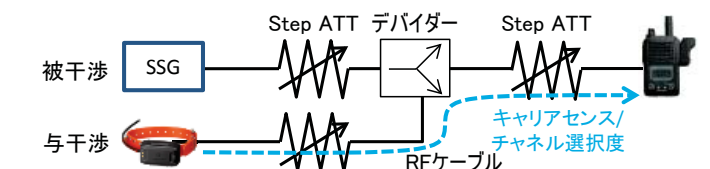
図4-20 測定構成
