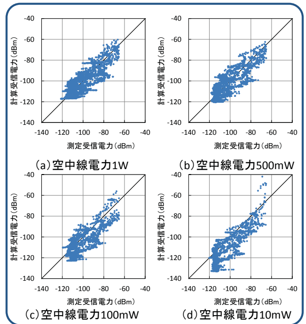
図4-15 測定受信電力と計算受信電力の相関
