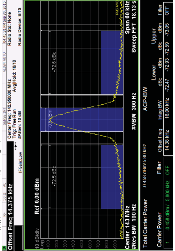
[1-2] 4値FSK 1Wチャネル間隔6.25kHz 離隔周波数14.375kHz 帯域16.0kHz (隣接システムへの漏えい電力)
