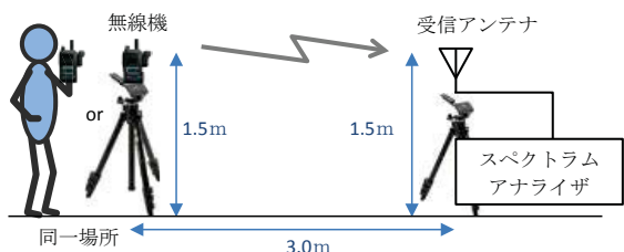
図4-18 測定構成
