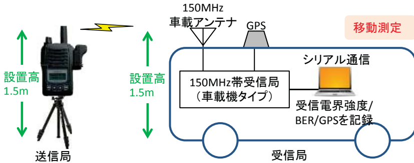
図4-13 測定構成図
