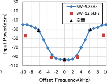
図4-30 キャリアセンス
