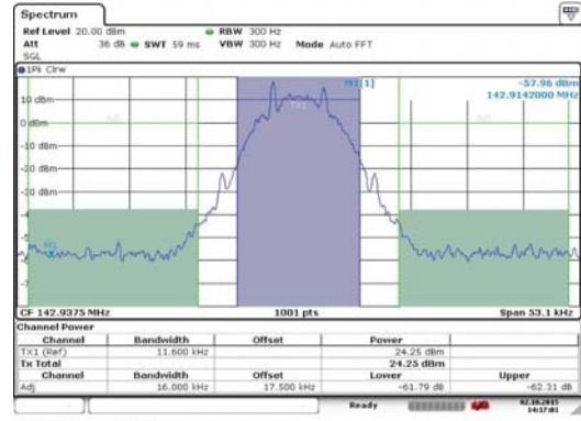
② 2CH結束利用時の隣接システムへの漏洩電力
