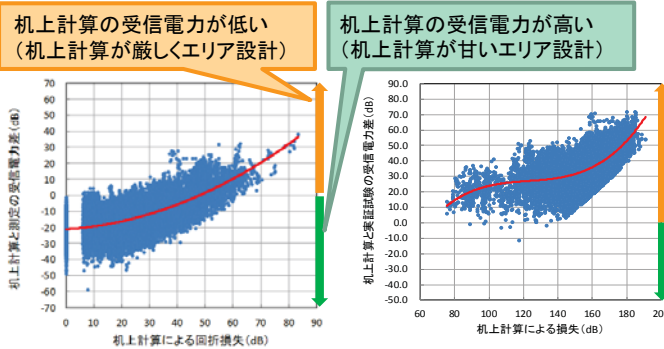
机上計算の回折損失と受信電力差の傾向 (多重回折損失計算)
