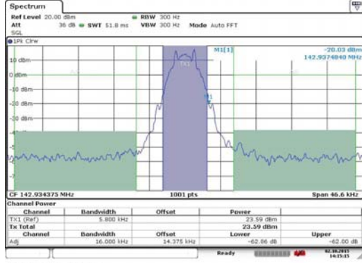
① 1CH利用時の隣接システムへの漏洩電力
