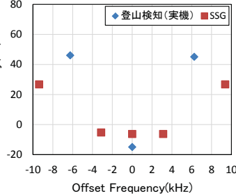
図4-28 隣接チャンネル選択度
