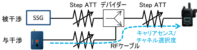
図4-26 測定構成
