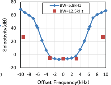
図4-31 隣接チャンネル選択度
