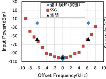
図4-27 キャリアセンス
