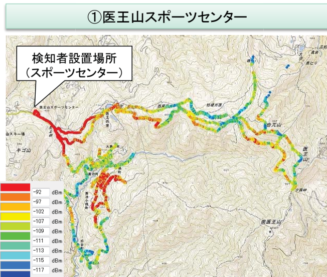
医王山スポーツセンターに設置した検知者端末における登山者端末からの受信電力マップ
