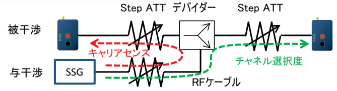
図4-29 測定構成
