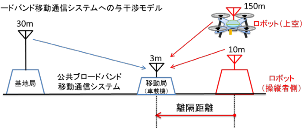
図参 2.3 公共ブロードバンド移動通信システムへの与干渉モデル
