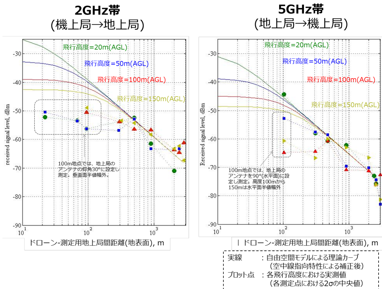
図参 5.2 測定結果
