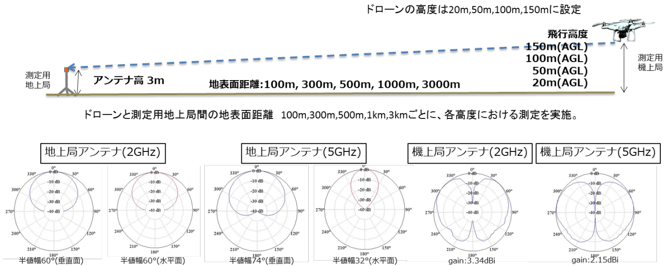
図参 5.1 測定条件
