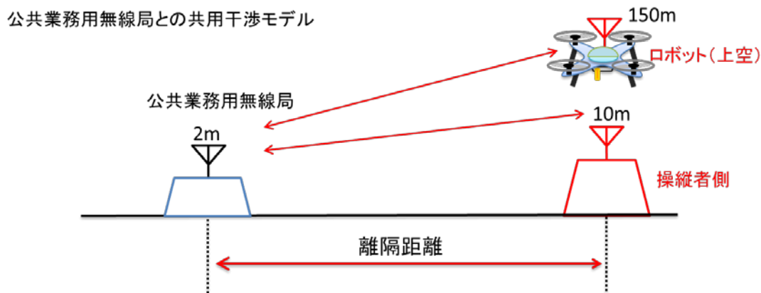
図参 2.5 公共業務用無線局との干渉モデル
