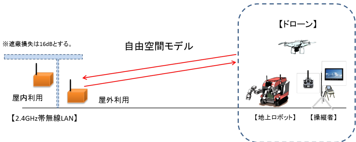
図 4.1 5GHz 帯無線 LAN との共用検討モデル
