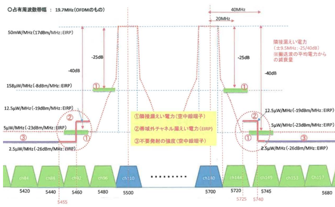
図参 1.1 5GHz 帯無線 LAN 共用検討諸元
