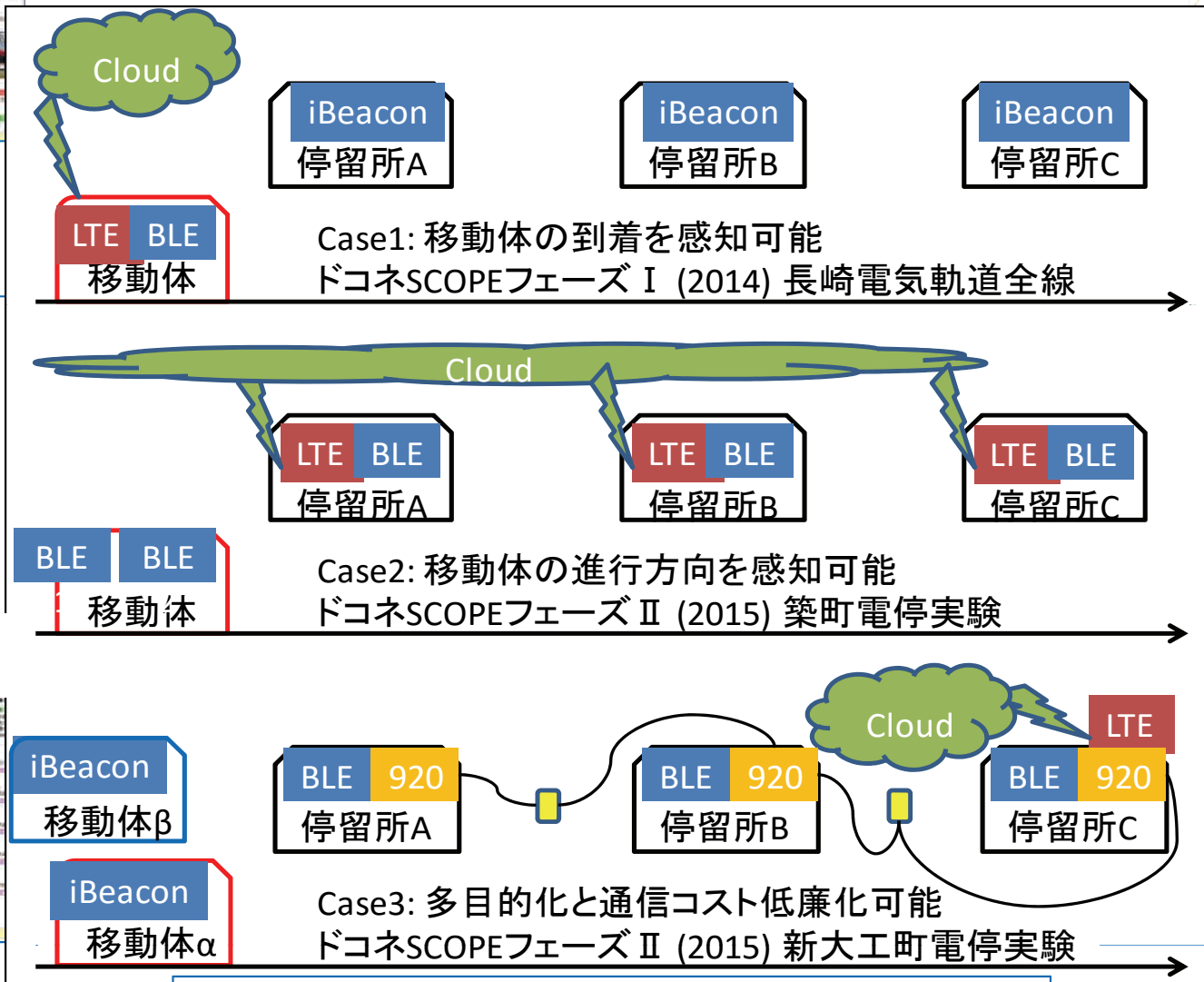
<平成26年度～平成28年度> 社会実験：ビーコンによる移動者支援ナビゲーション
