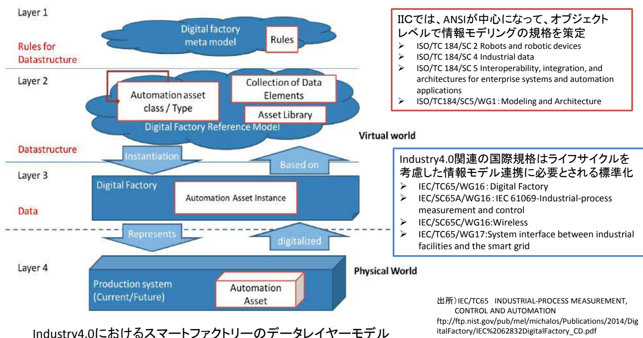
図表 3-6 欧米によるスマートファクトリーの標準化
