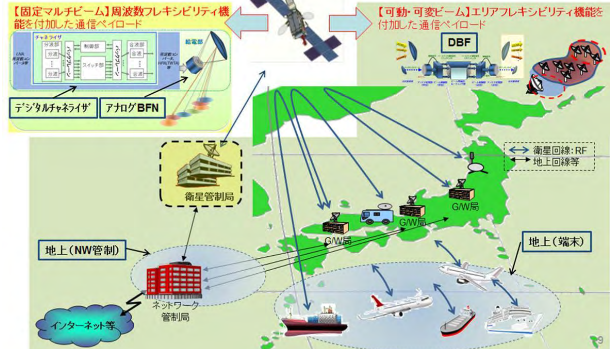
衛星通信システム全系
