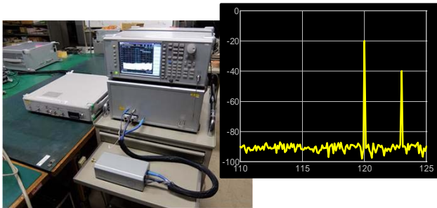
110GHz~140GHzスペクトラム測定系
