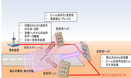
図2-2-23 リニアセル・センサーネットワークの検知性能向上のための研究開発
