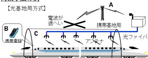
図3-1-19 電波遮へい対策事業
