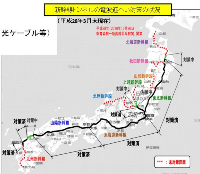
図3-1-19 電波遮へい対策事業
