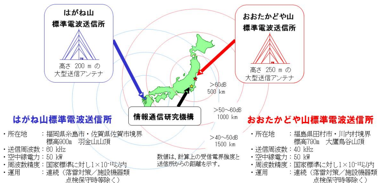
図3-1-15 標準電波の発射
