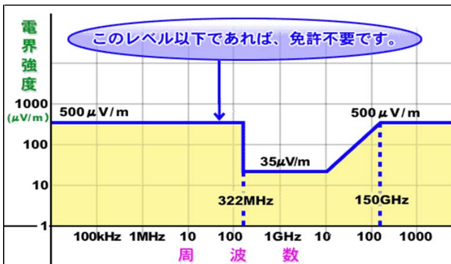
図3-2-8 微弱無線局の3mの距離における電界強度の許容値
