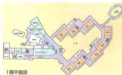
2階平面図
