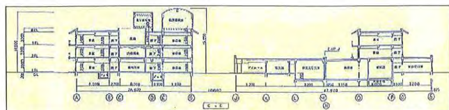
断面図
