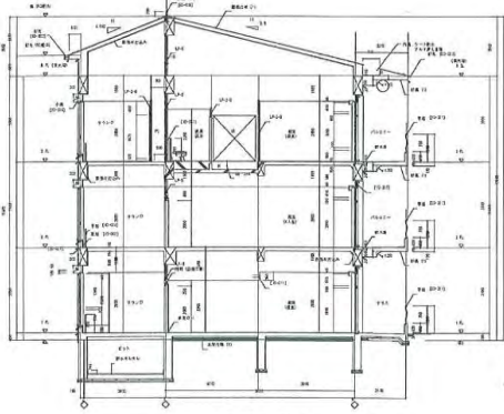
断面図
