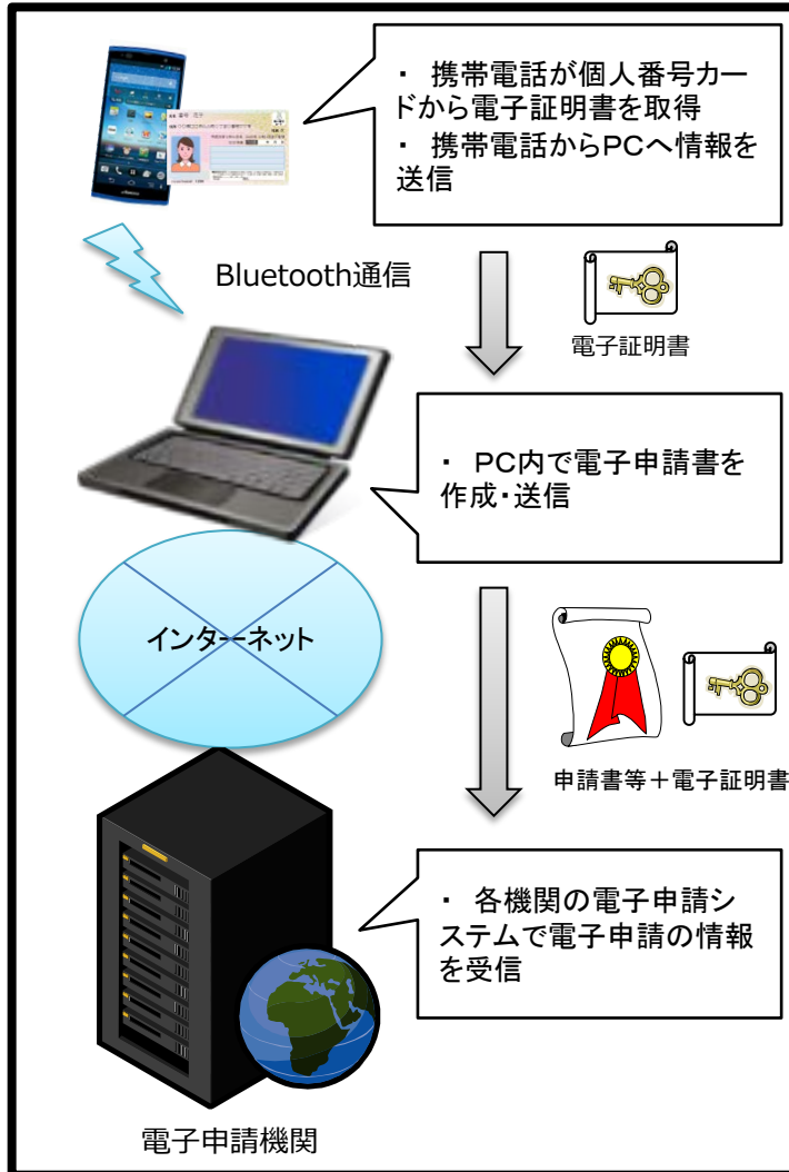
【方式1】携帯電話をICカードリーダーとして使用し、携帯電話とPCを連携させる
