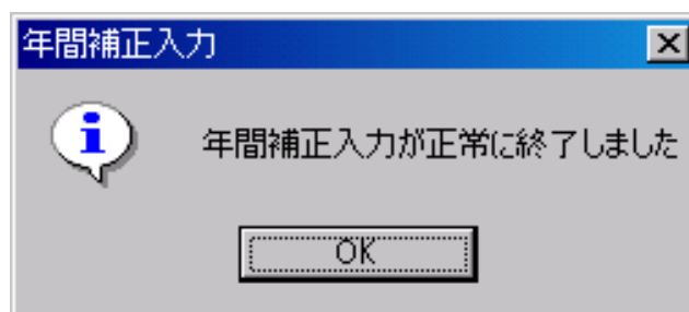
図 2.12.1-3 実行結果
