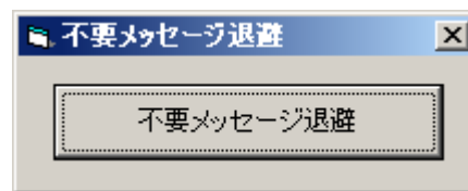
図 2.13.1-1 メイン画面
