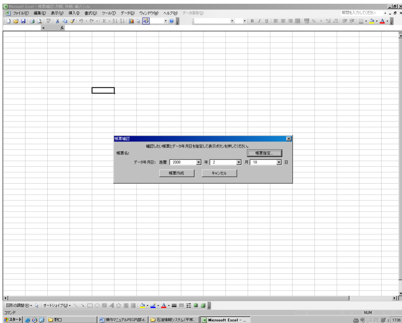
図 2.7.1-1 メイン画面
