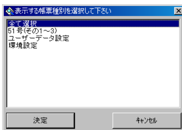
図 2.4.1-1 メイン画面
