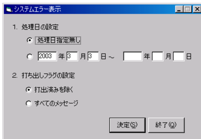
図 2.5.1-1 メイン画面
