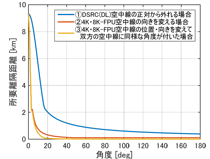
空中線の向きを考慮した所要離隔距離
