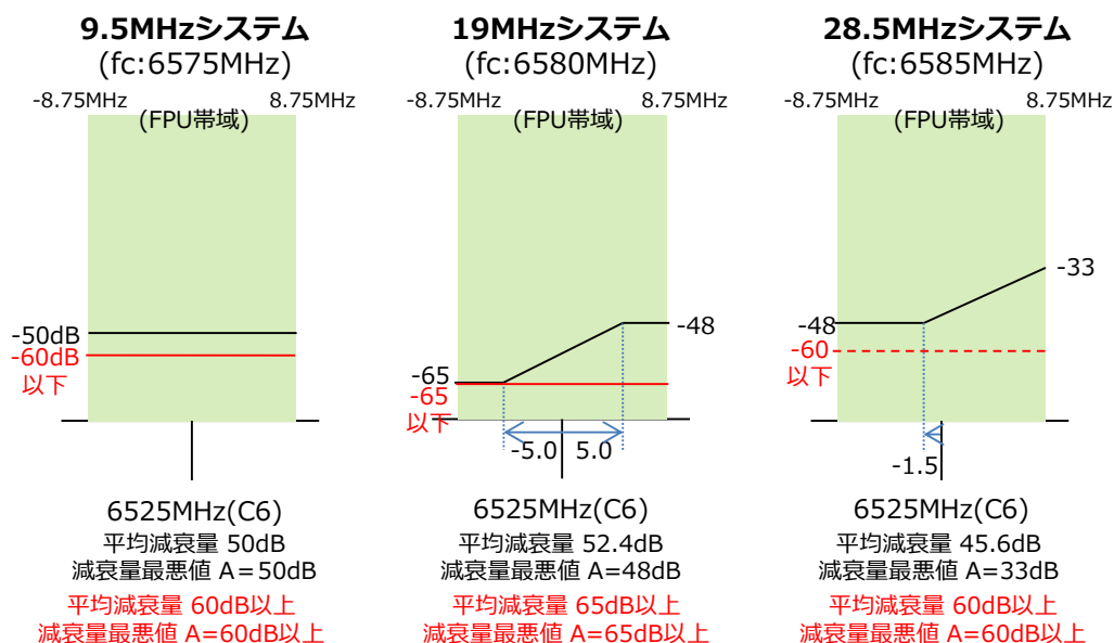
図 1 7 ㊦ F P U 帯域内（チャンネル C6）への漏洩電力
