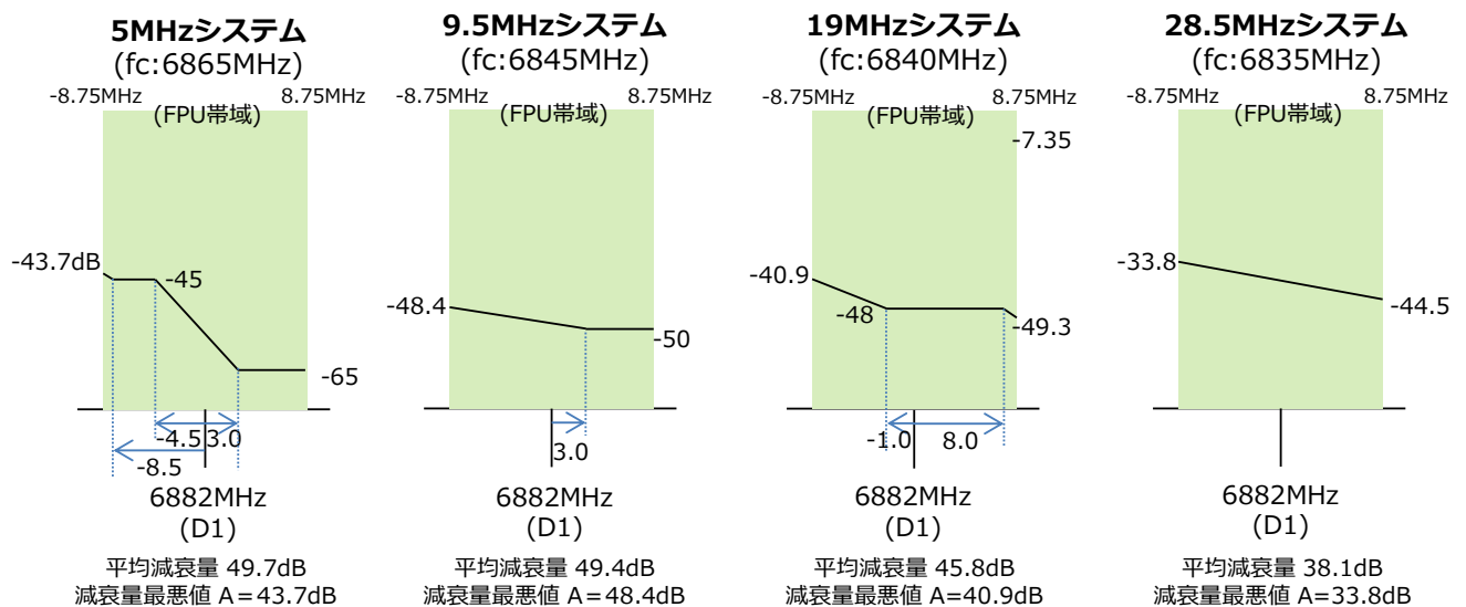
図 1 6 ㊦ F P U 帯域内（チャンネル D1）への漏洩電力
