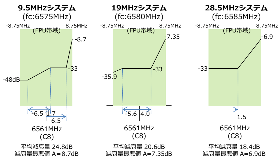
図 1 5 ㊦ F P U 帯域内 (チャンネル C8) への干渉波漏洩電力
