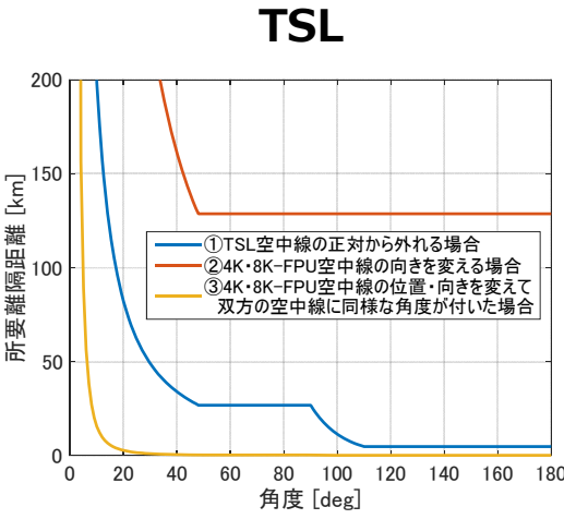
固定中継（高品質伝送）モデルの場合（最悪値の場合）
