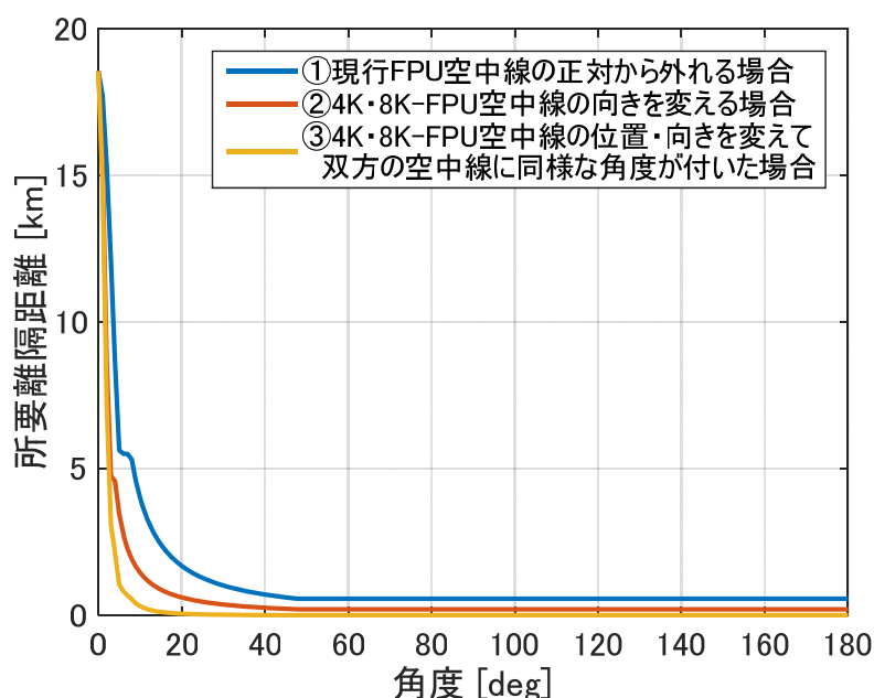
図 3. 1 5 空中線の向きを考慮した所要離隔距離（現行 F P U と隣接チャンネルで、固定中継（高品質伝送）モデルの場合）
