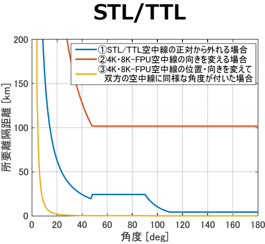
IF伝送方式で、固定中継（高品質伝送）モデルの場合（最悪値の場合）
