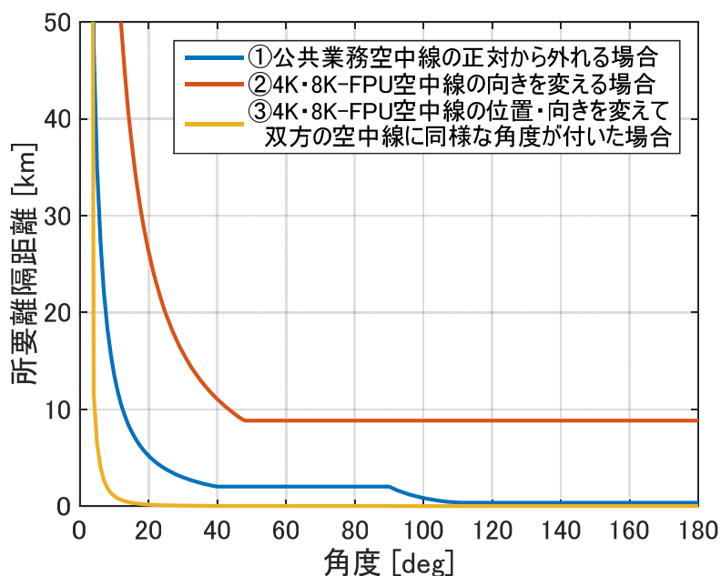
図 3. 7 空中線の向きを考慮した所要離隔距離（28.5MHz システムと C8 チャンネルが隣接で、固定中継（高品質伝送）モデルの場合）
