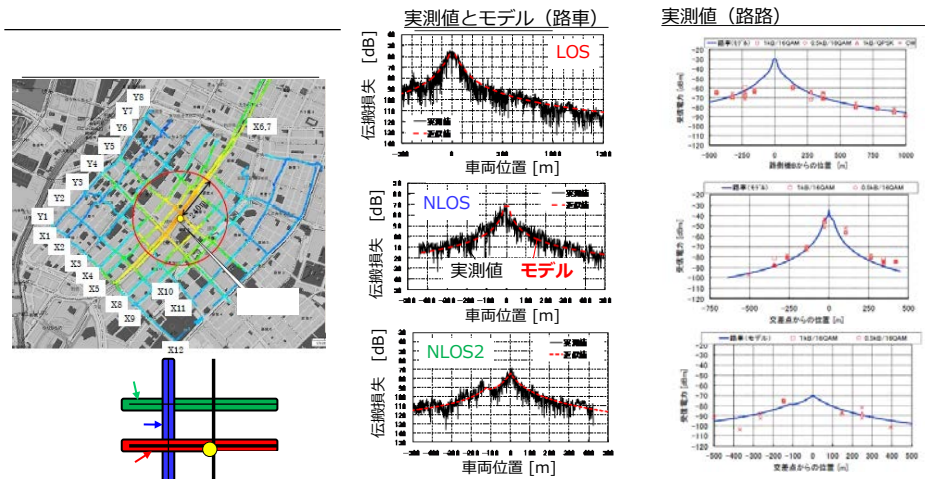
図 17 伝搬損失モデル
