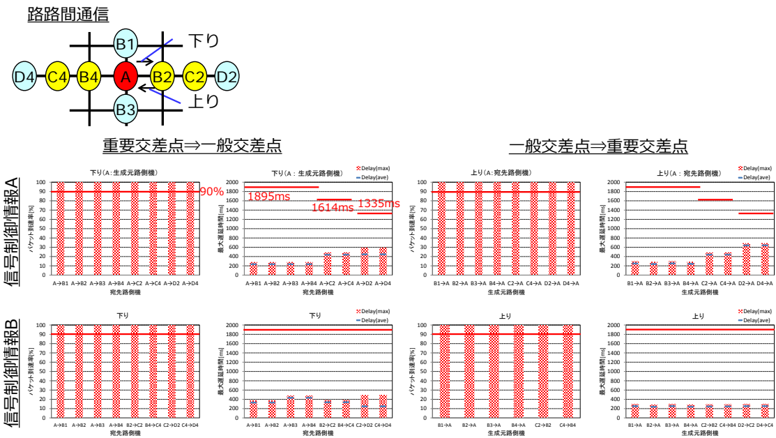
図 29 シミュレーション結果 (パターン8)
