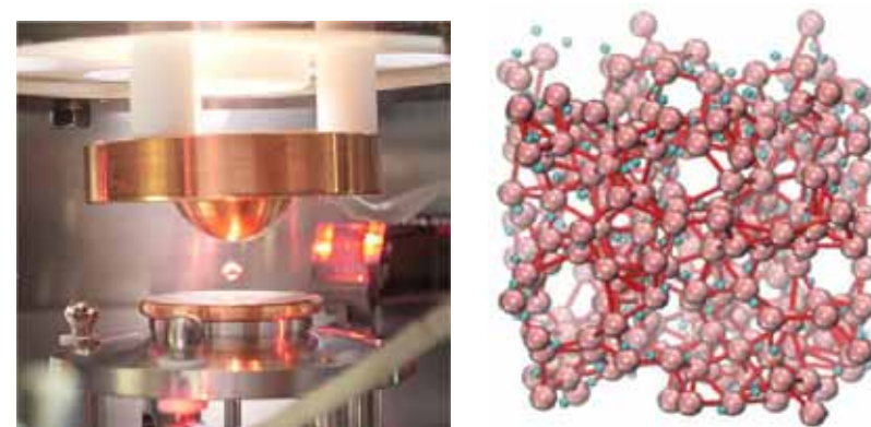
(左) : 静電浮遊法で浮遊する試料 (右) : SPring-8で得られたデータから解析した溶融ホウ素の電子構造
