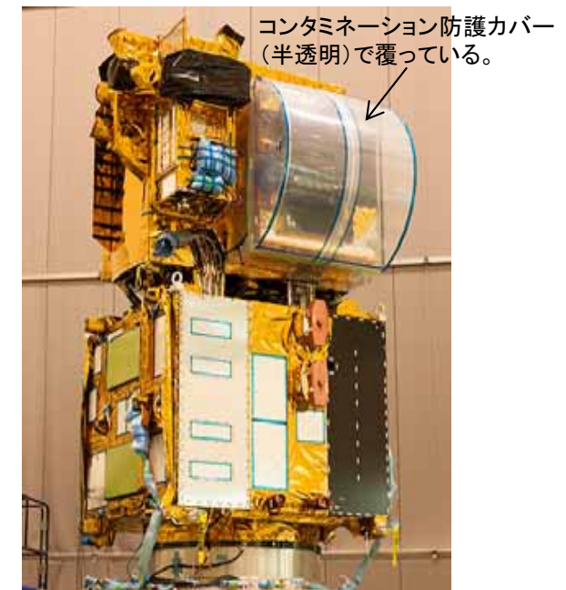
GCOM-C外観
