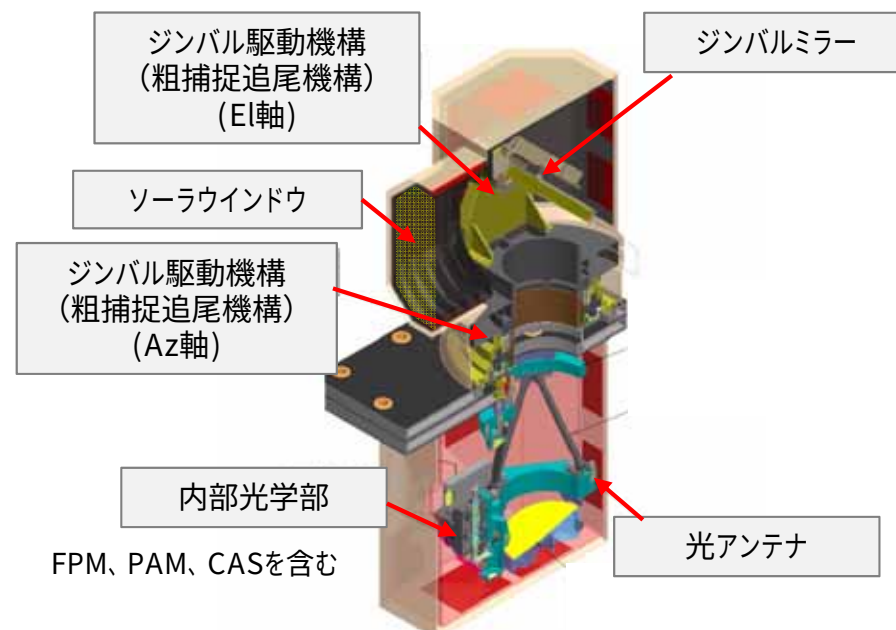
光データ中継衛星搭載光衛星間通信機器の内部
