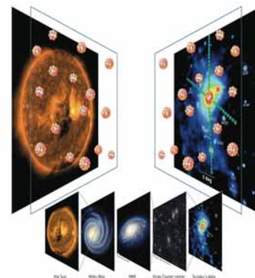
おとめ座銀河団（右上）で計測された元素組成が太陽（左上）と同じであることがわかったことから、宇宙の様々なスケール（下）での元素組成も太陽と同じと考えられる。
