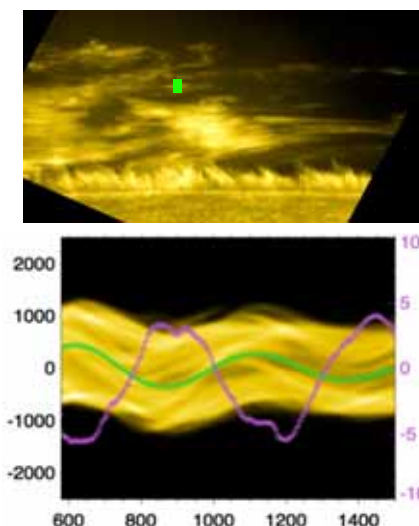
緑色の領域のプロミネンス震動を、「ひので」とIRISで同時観測し、波動散逸を同定した。
