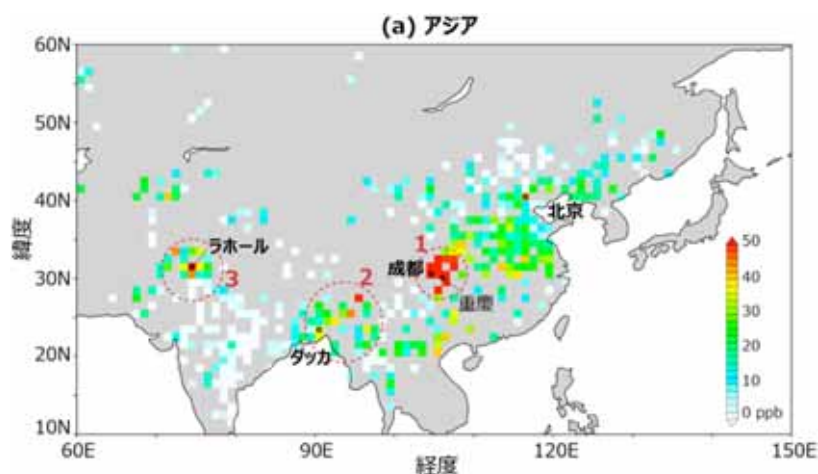
GOSATによる人為起源メタン濃度 (ppb)
