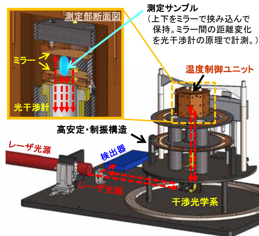
技術検証用のプロトタイプモデル
