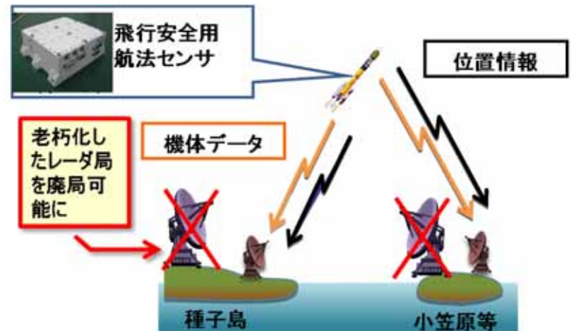
航法センサを用いた飛行安全管制
