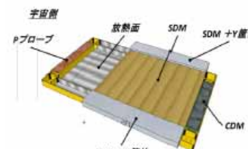
KASPERセンサ
