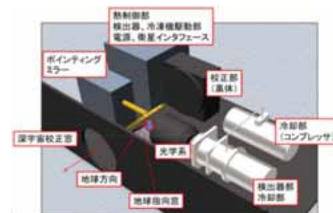
衛星搭載型赤外線センサ イメージ図 (出典：宇宙開発利用部会防衛省説明資料)
