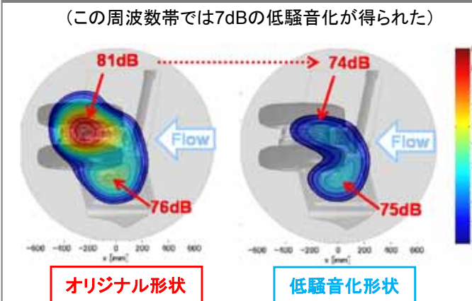
音源計測による車間ポラスフェアリングの効果の評価(2kHz)
