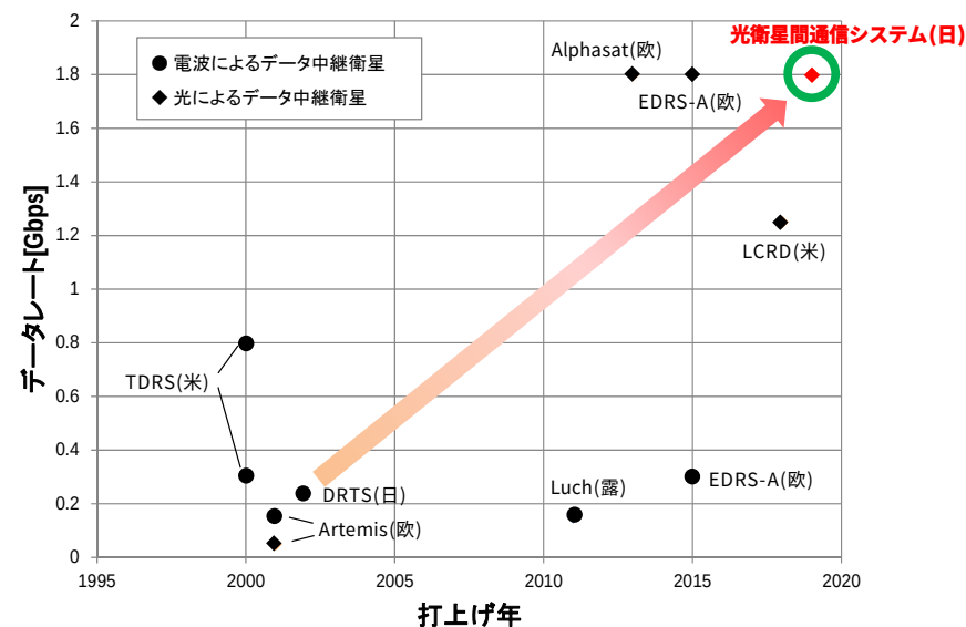
データ中継システムの性能比較
