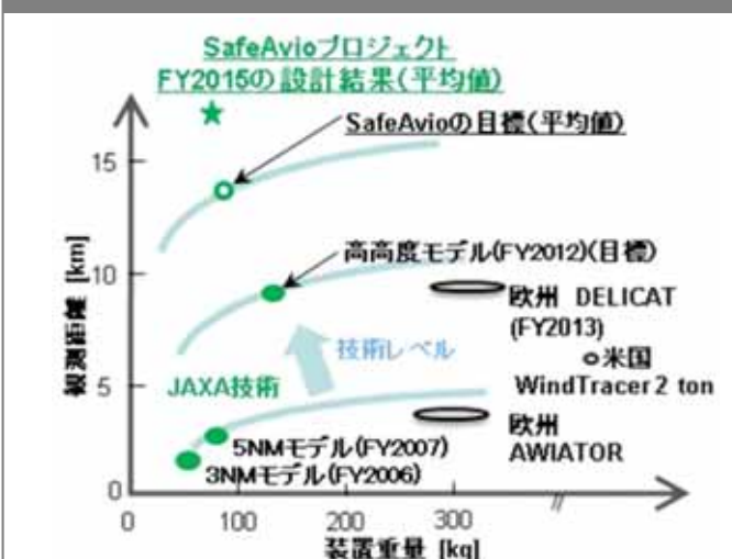
乱気流検知装置の重量と観測距離比較
