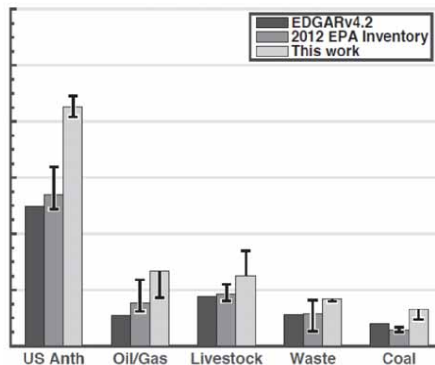
北米メタン排出
