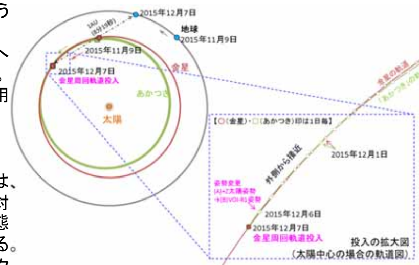
金星周回軌道投入時の軌道図（太陽中心）
