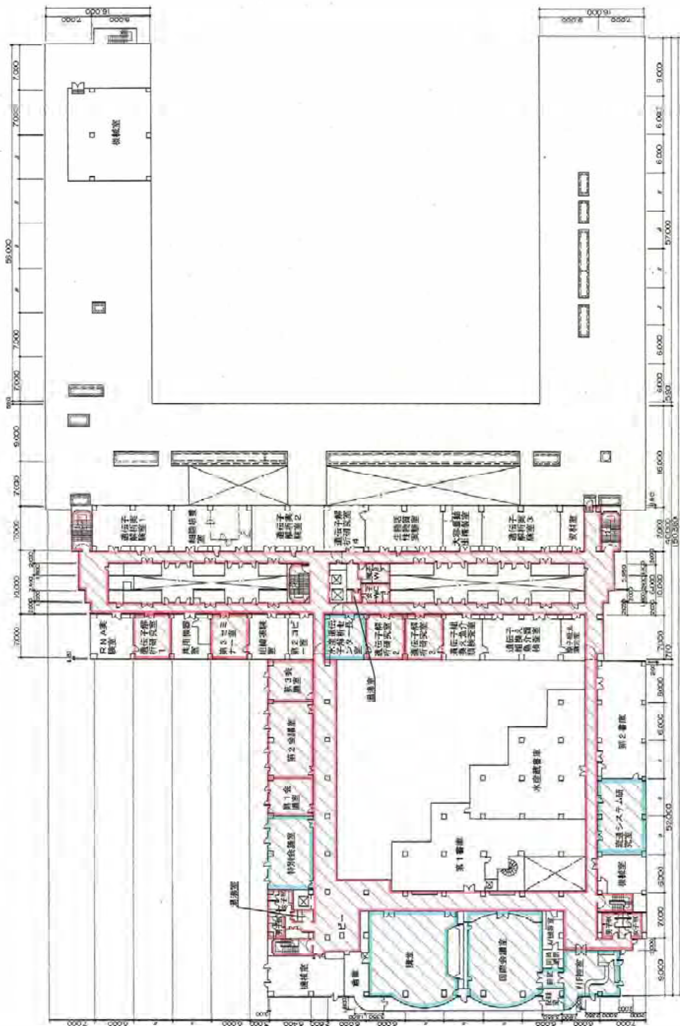
3 階平面図
