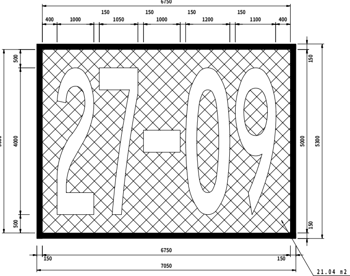
(N-2・3・4 (西側) 誘導路用停止位置案内標識用詳細図)
