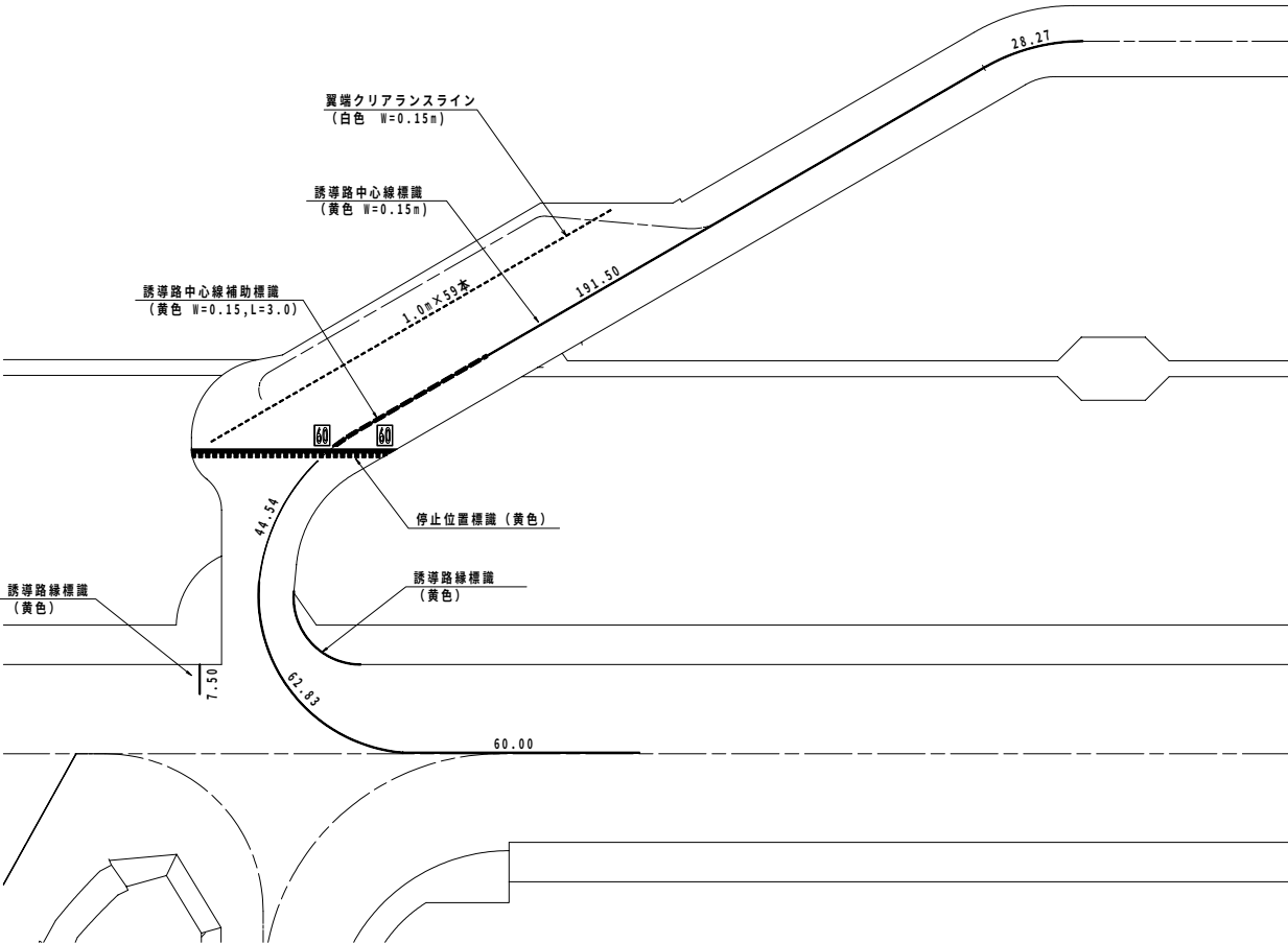
N-1 誘導路 S=1:1000
