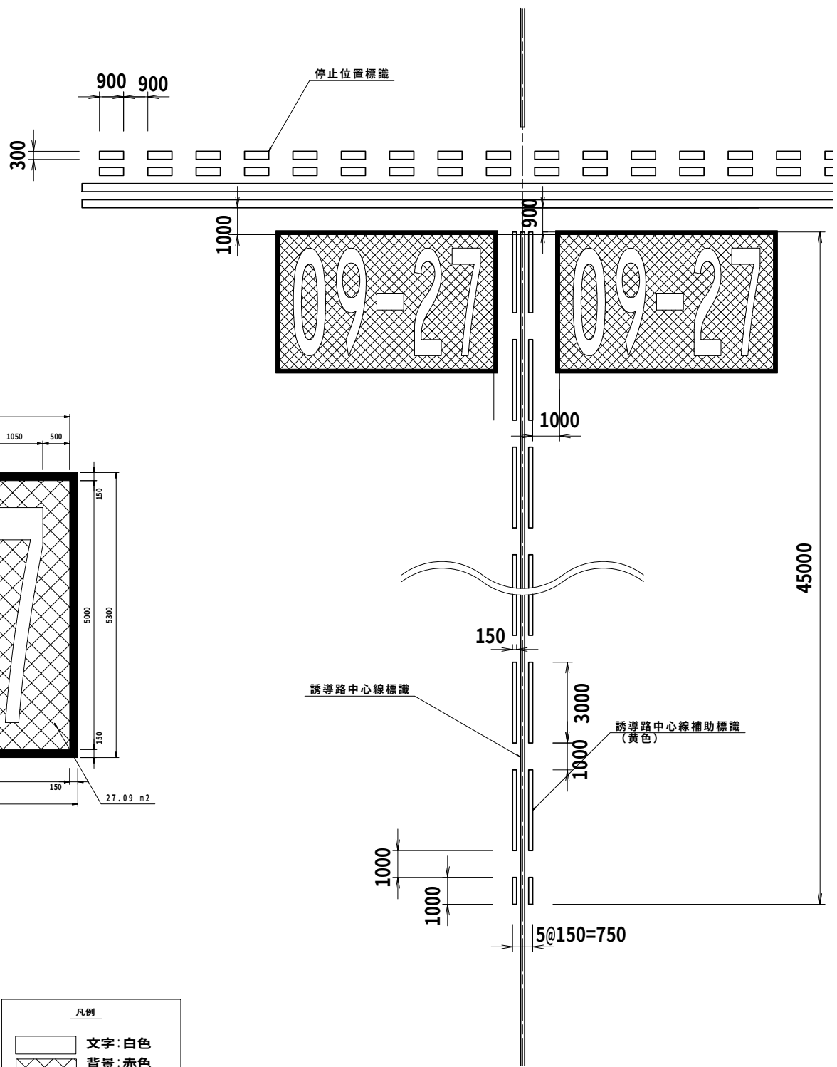
誘導路中心線標識等詳細図
