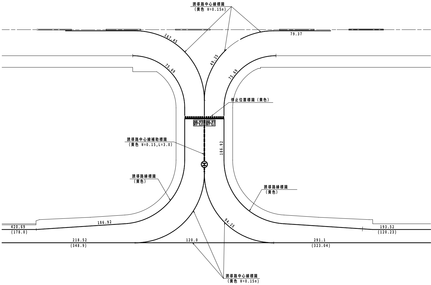
S-3 誘導路 S=1:1000
