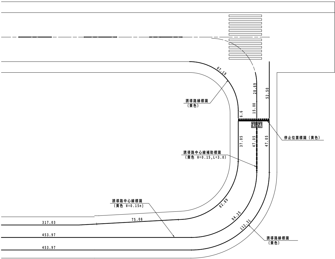
S－8 誘導路 S=1:1000
