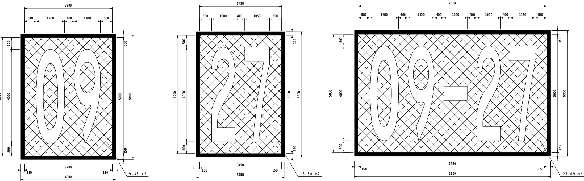
(N-2・3・4 (西側) 誘導路用停止位置案内標識用詳細図)
