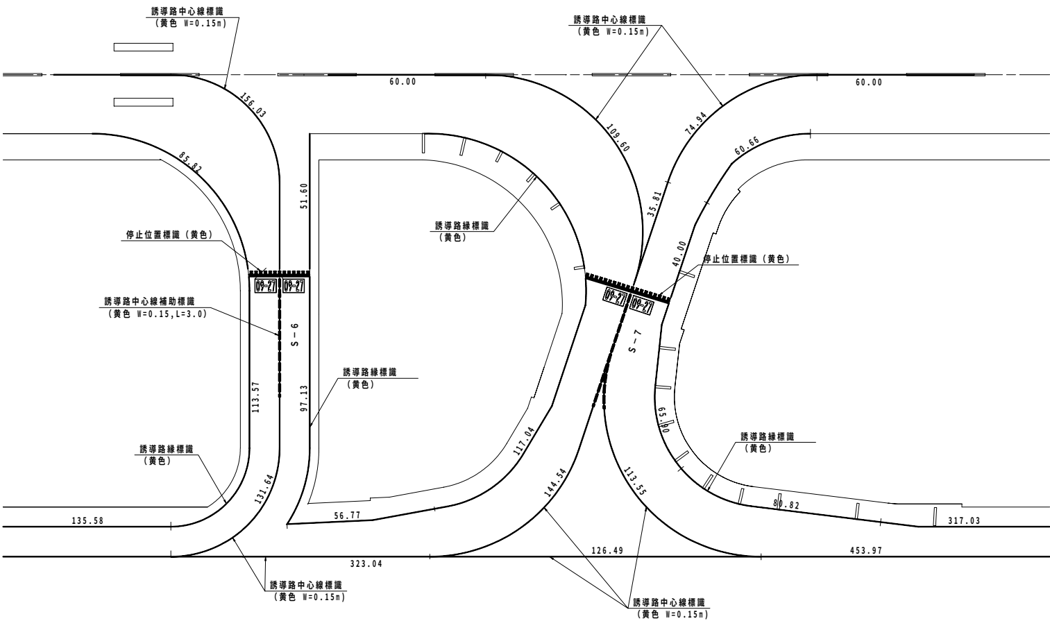
S－6，S－7 誘導路 S=1:1000
