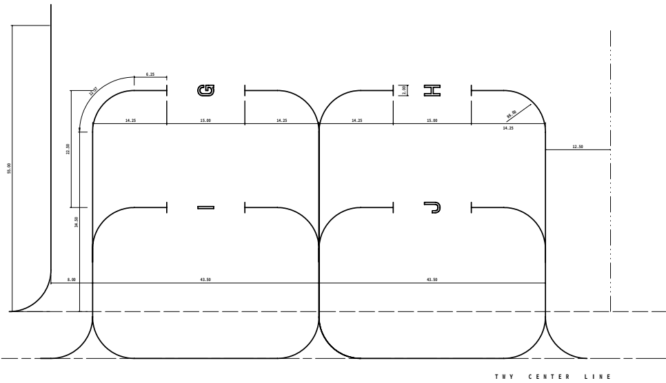
北側エプロン標識図 S=1:500
