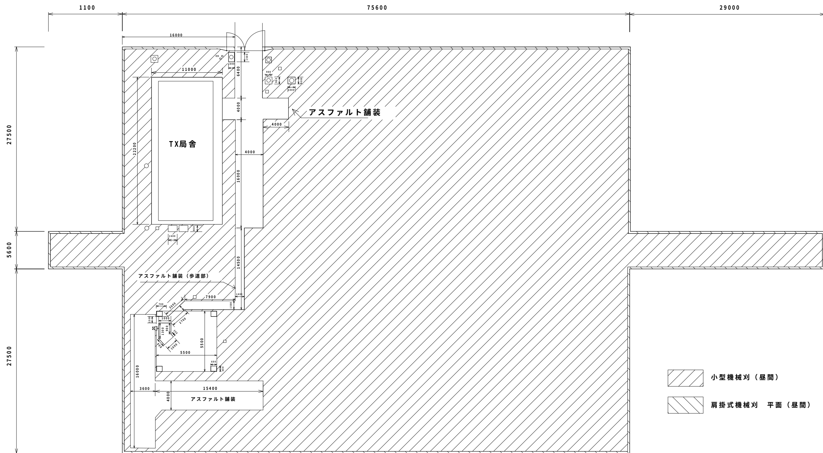
TXサイト敷地平面図 (S = 1/350)
