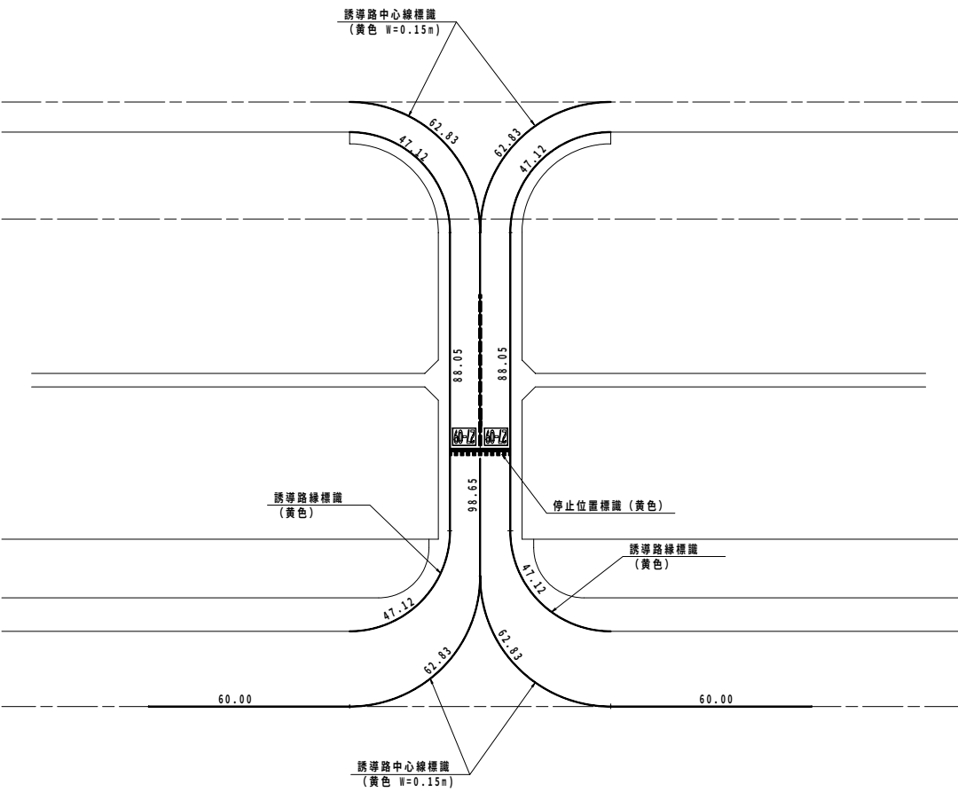
停止位置標識 S=1/200
