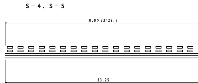
停止位置標識 S=1/20
