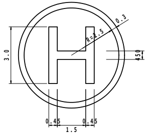
ヘリパッド標識 S=1/100
