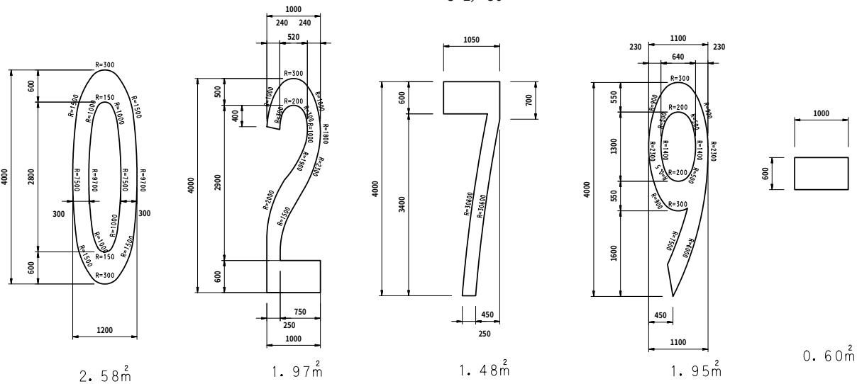
停止位置案内標識
