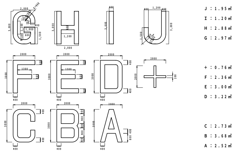
1 番 SPOT、北側エプロン文字詳細 S=1:100
