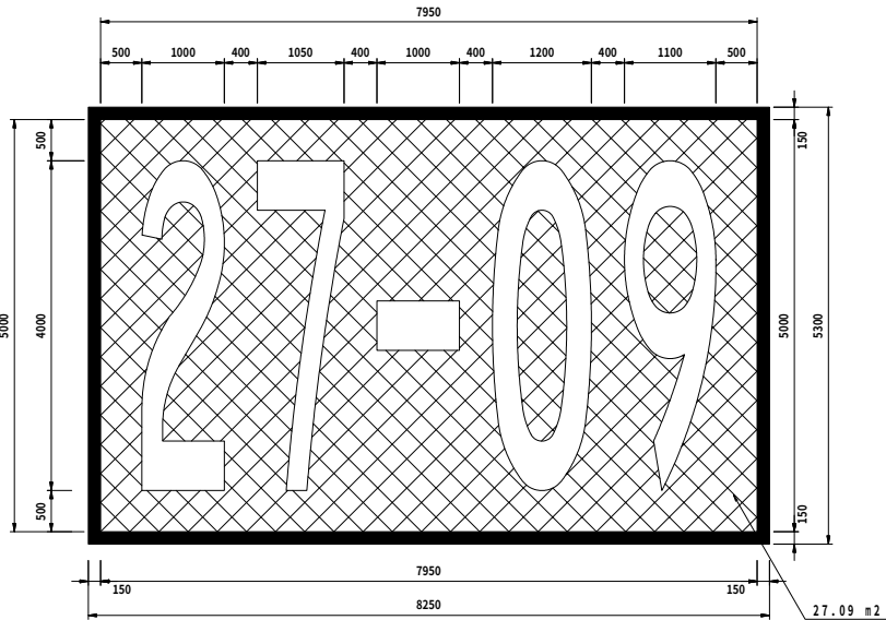
(N-4 (東側) 誘導路用停止位置案内標識用詳細図)
