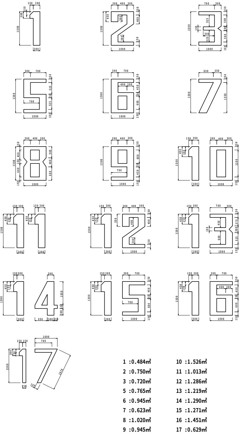
17° ロンスポット番号 S=1:50
