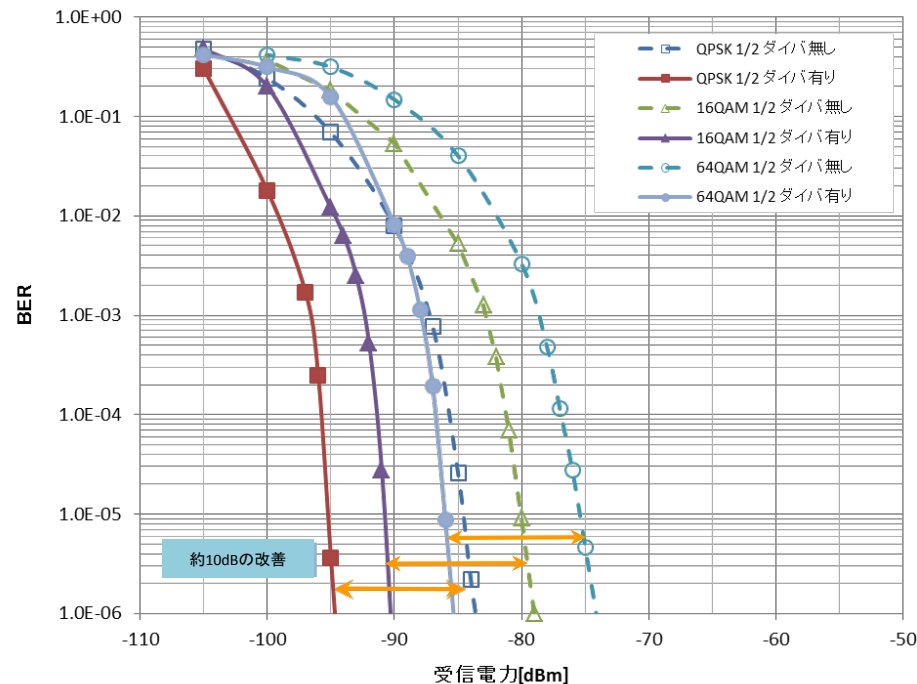
【COST 207 Rural AreaモデルのBER特性】
