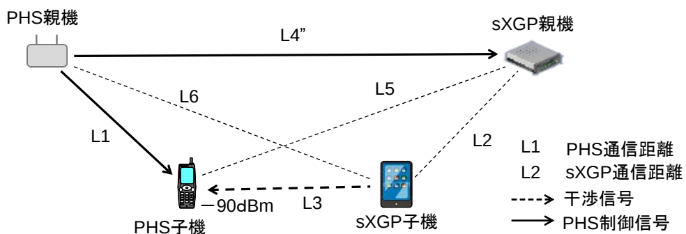
図 参 6 - 4 自営 PHS 方式制御チャネルに対する sXGP 子機からの干渉
