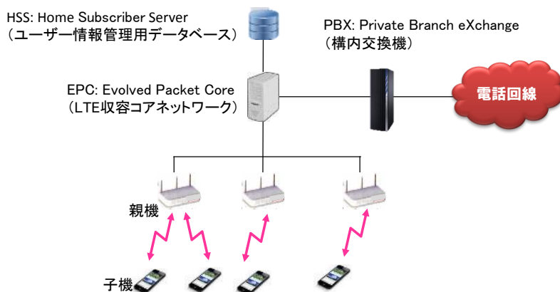
図 1. 3-3 sXGP 方式のシステム装置構成
