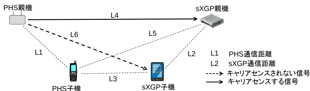
図 参 6 - 1 PHS 親機から送信される電波のキャリアセンス
