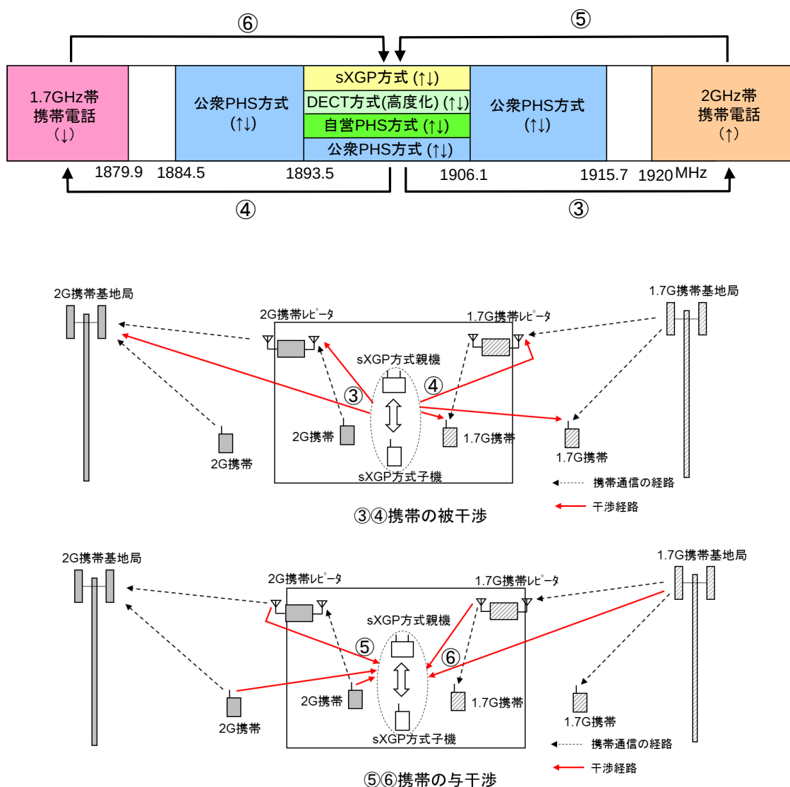
図 4. 4-1 携帯電話との周波数配置及び干渉経路の組合せ
