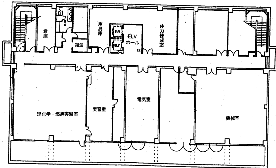
地下1階
