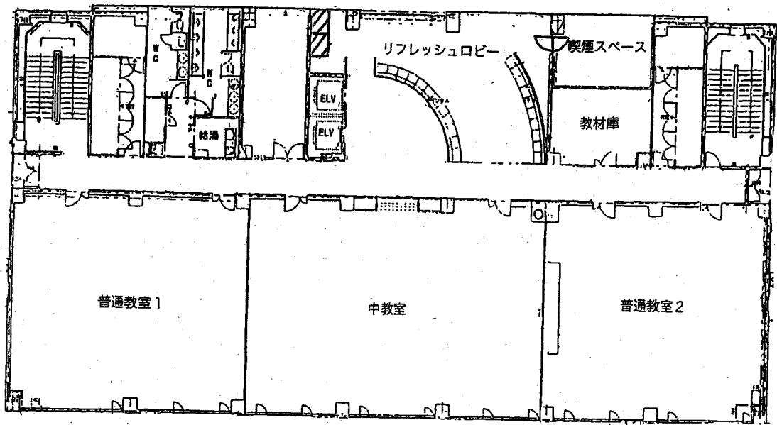
3 階
