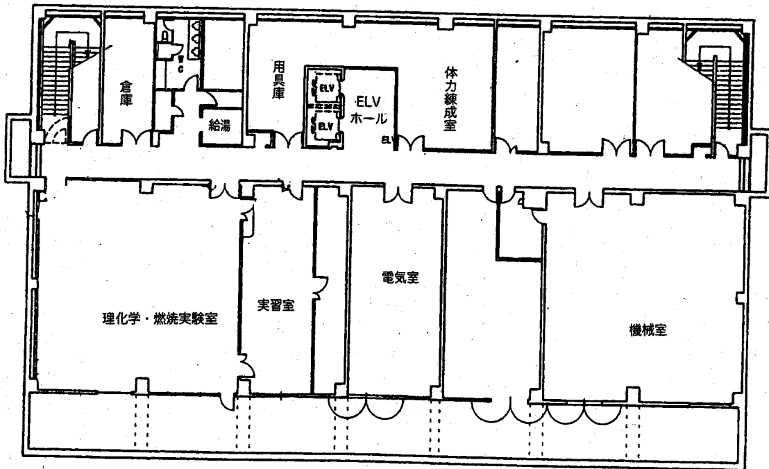
地下1階
