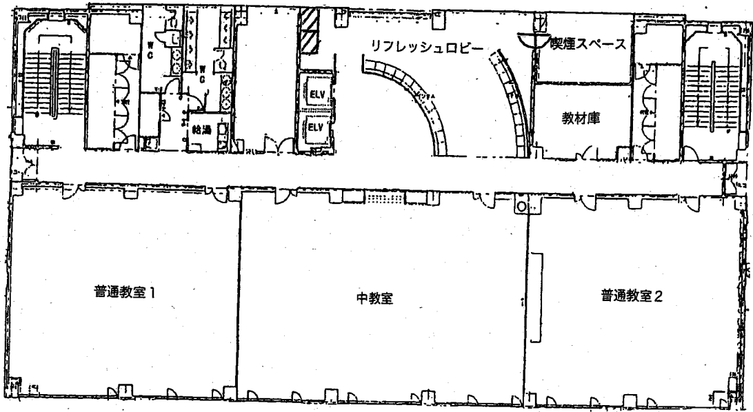
3 階
