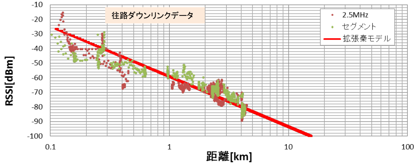
大手町-虎ノ門-千駄ヶ谷_移動データ_往路_DL距離 vs RSSI
