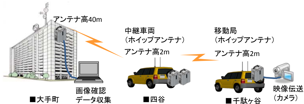
基地局(3素子八木アンテナ)
