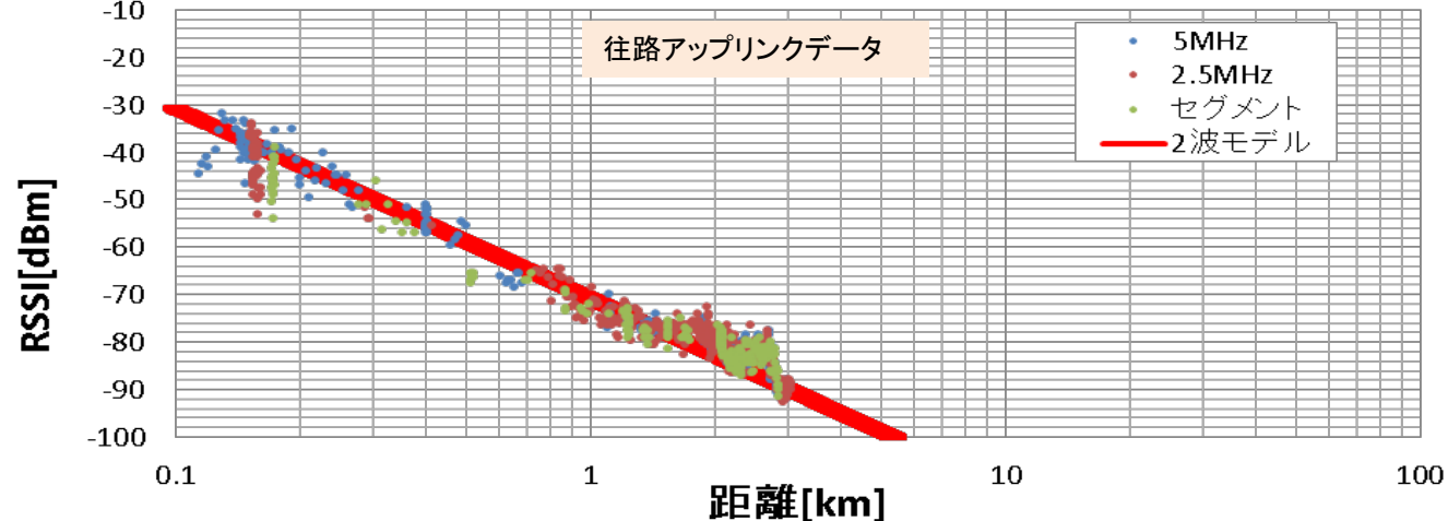
武蔵五日市-乙津_移動データ_往路_UL 距離 vs RSSI
