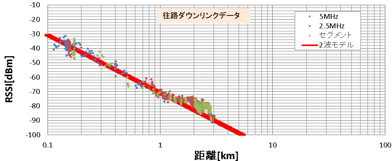
武蔵五日市-乙津_移動データ_往路_DL 距離 vs RSSI
