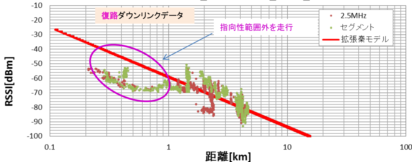
大手町-虎ノ門-千駄ヶ谷_移動データ_復路_DL距離 vs RSSI
