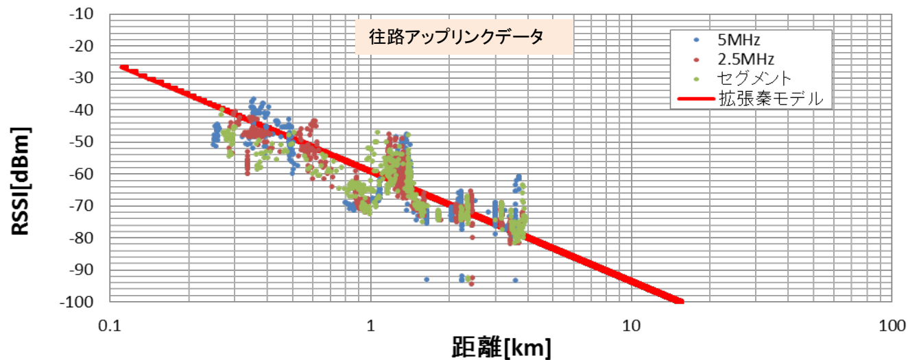
大手町-千鳥ヶ淵-新宿区富久町_移動データ_往路_UL 距離 vs RSSI
