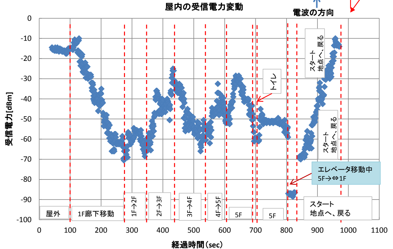
ビル: 79.4m(W) × 46.8m(D) × 22.6m(H)
