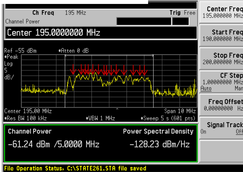
千鳥ヶ淵受信電力波形
