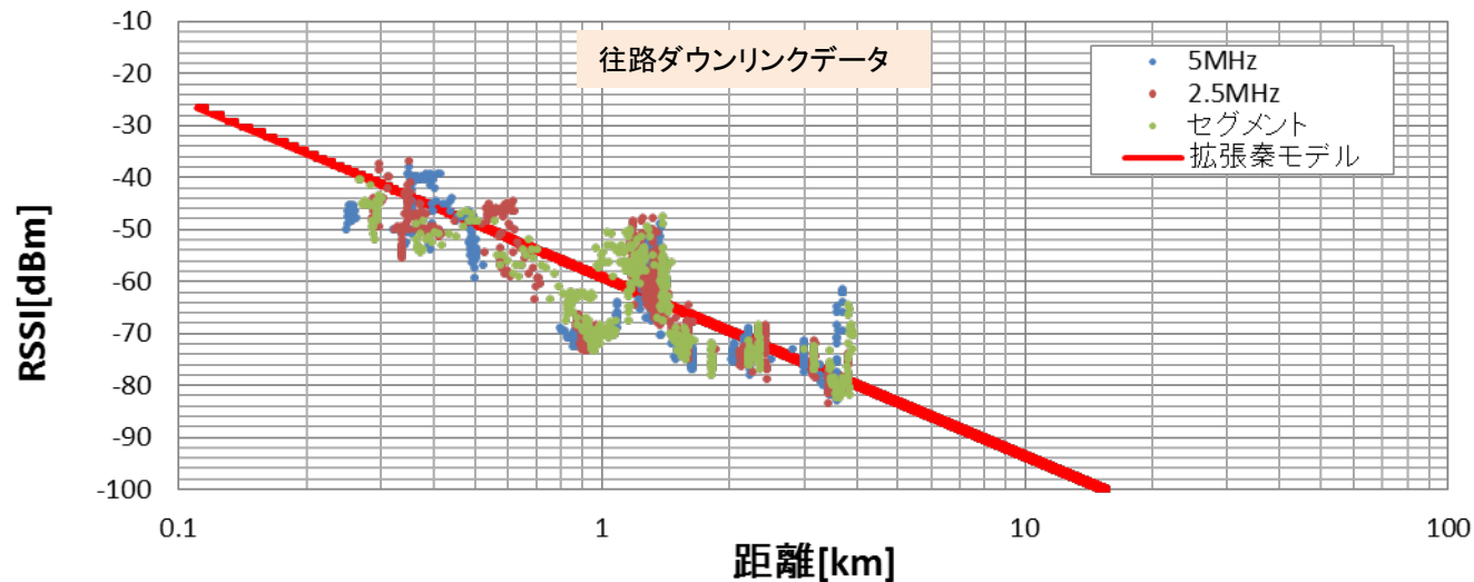
大手町-千鳥ヶ淵-新宿区富久町_移動データ_往路_DL 距離 vs RSSI
