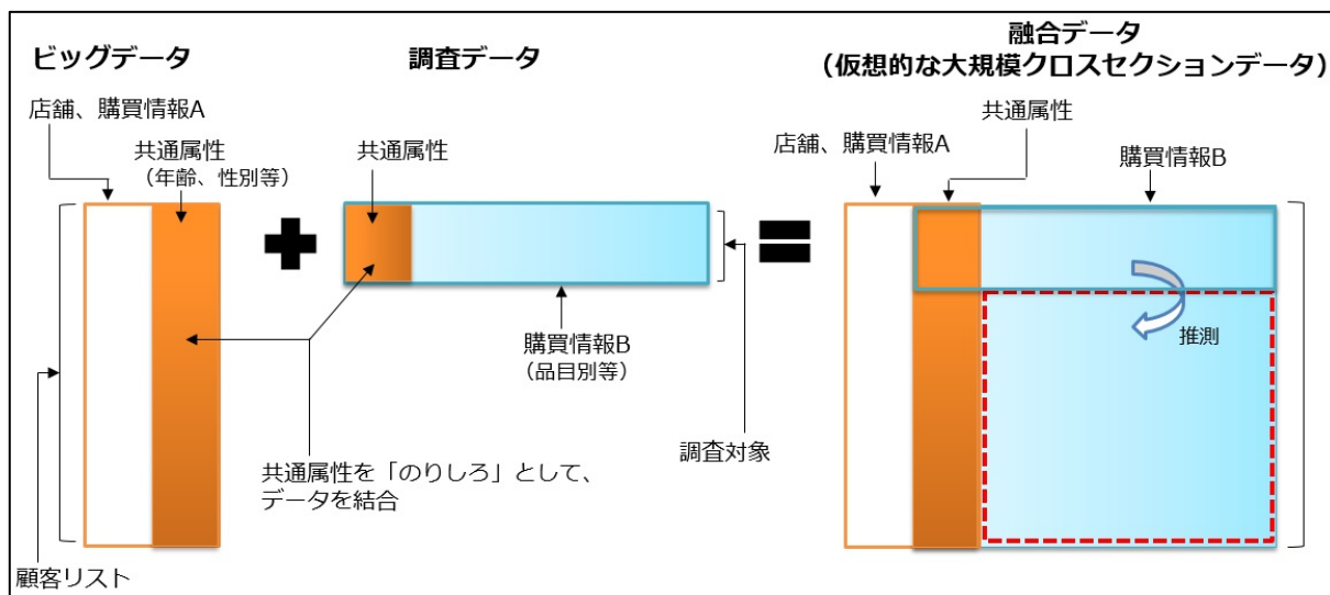
図Ⅱ-10 ビッグデータのバイアス補正・データ融合の概念図
