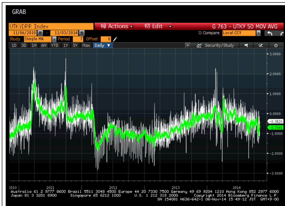
図 A-1 Bloomberg 上で配信されている東大日次物価指数
