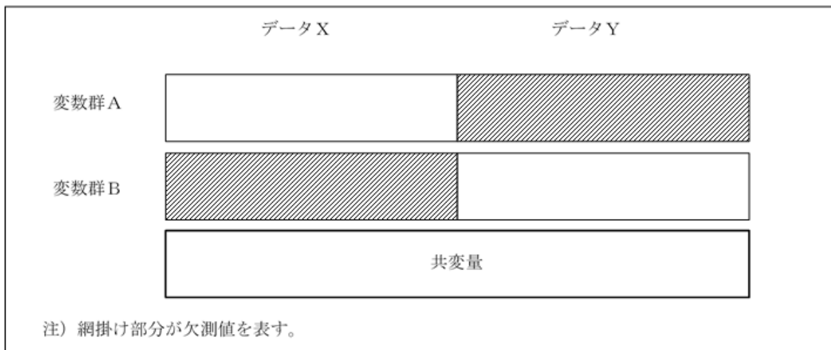
図Ⅱ-9 欠測値推定の基本概念図
