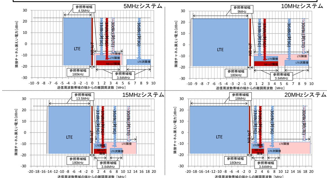
図2. 2-2 NB-IoT 移動局の隣接チャネル漏えい電力
