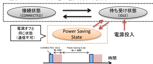
図2. 1-1 eMTCとNB-IoTに共通した主要技術
