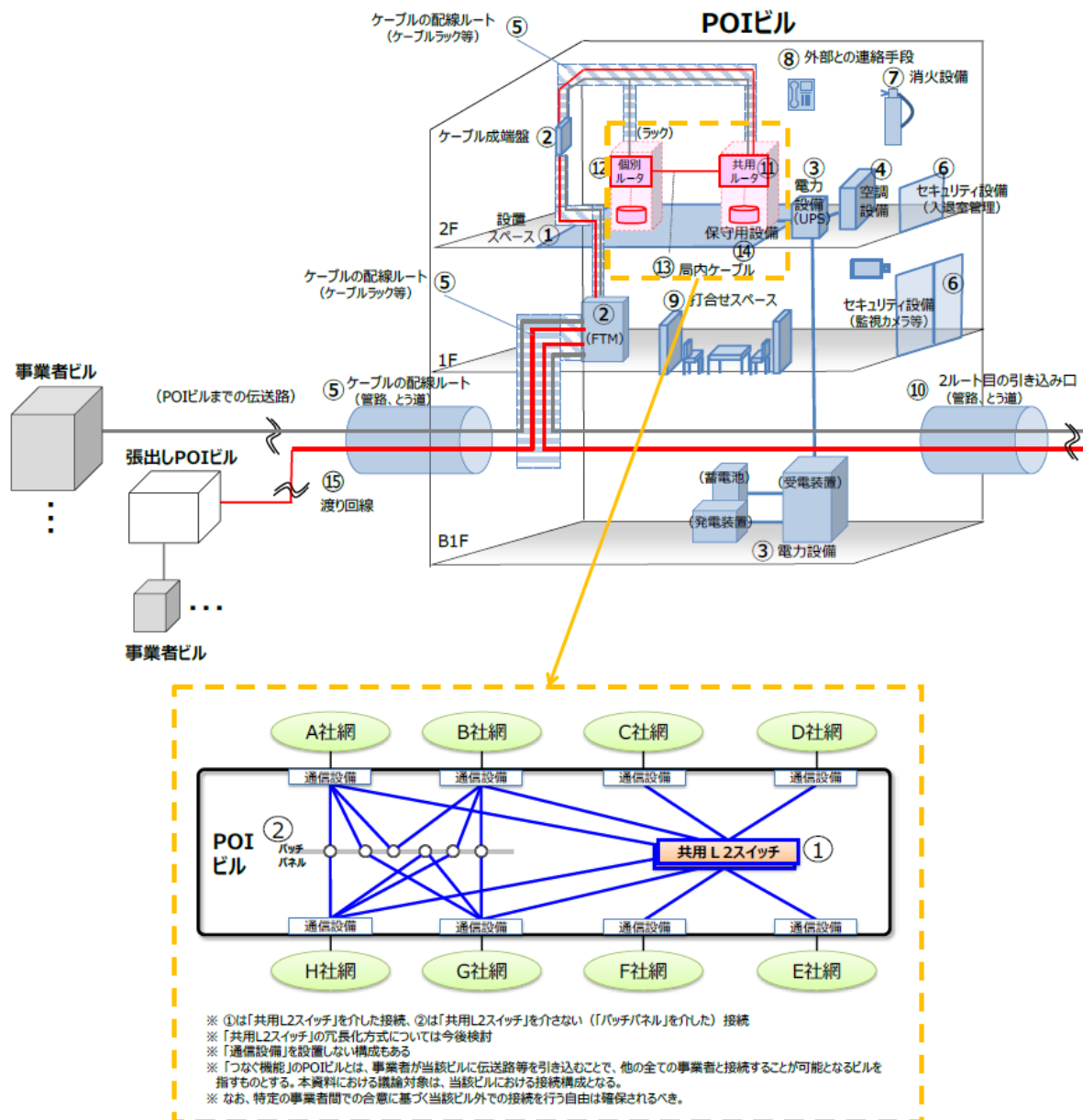
図 1.2.3 事業者間で協議された「繋ぐ機能 POI ビル」内の設備構成
