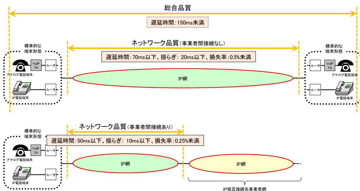
図 4.2.1 0AB-J IP 電話用設備に関する移行後の音声品質に係る技術的条件
