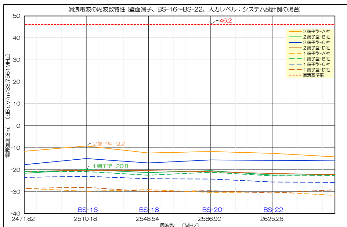
図 20 設計例に従って換算した場合の壁面端子の漏洩電波の最大電界強度(BS-16~BS-22)
