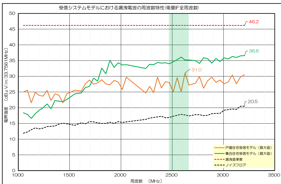
図 29 宅内配線モデルの周波数特性(各周波数の最大値)
