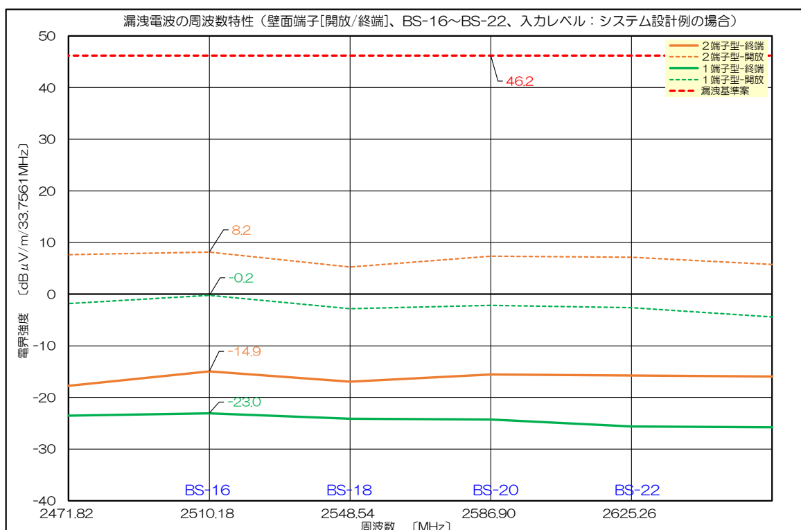
図 24 壁面端子(開放-終端比較)(BS-16~BS-22)
