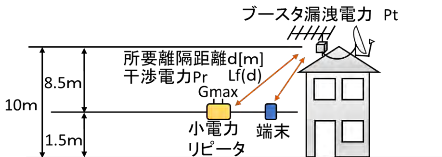
図 3.4.2-4 WiMAX 小電力レピータ・端末の干渉評価モデル（屋外） このモデルにおける干渉電力 P_r は以下の計算式で算出できる。
