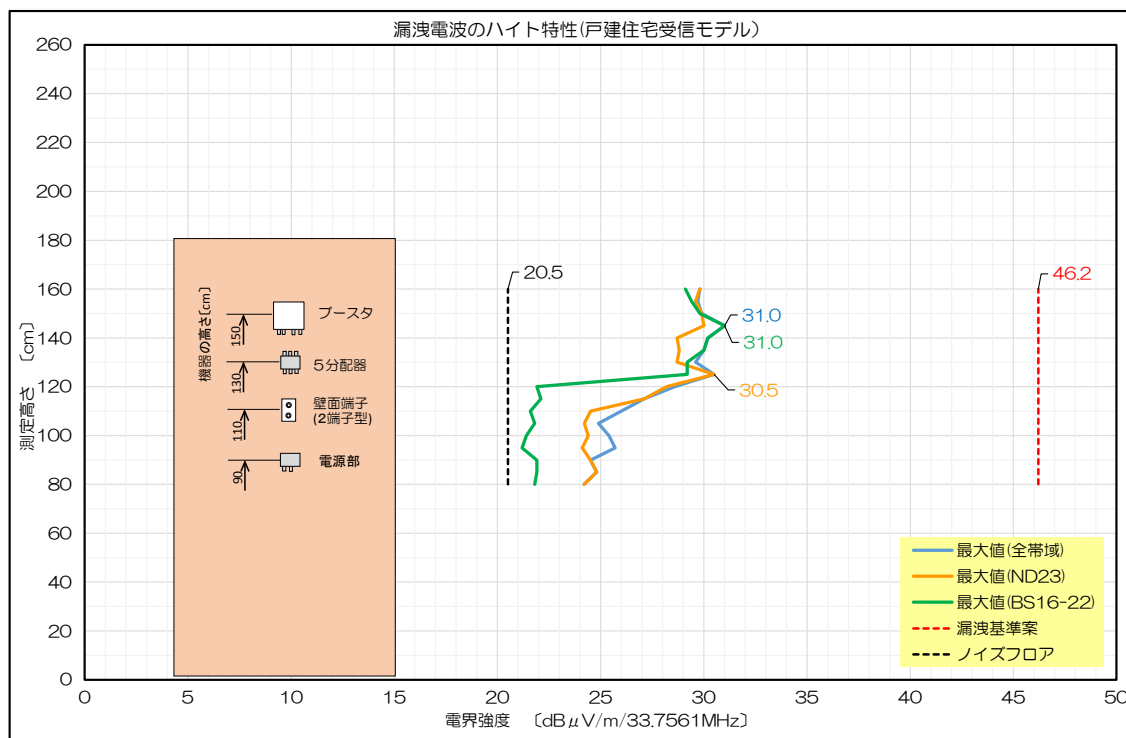
図 31 戸建住宅モデルの漏洩電界強度の高さ方向の分布
