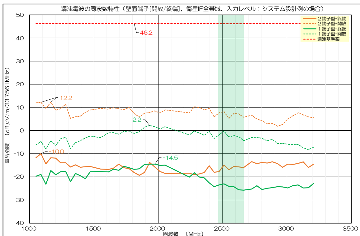
図 23 壁面端子(開放-終端比較)(各周波数の最大値)
