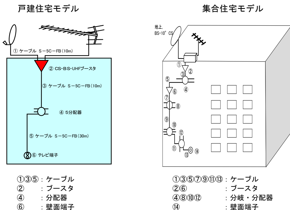
図 25 配線モデル (ARIB STD-B63 1.6 版 P.80 および P82 参照)
