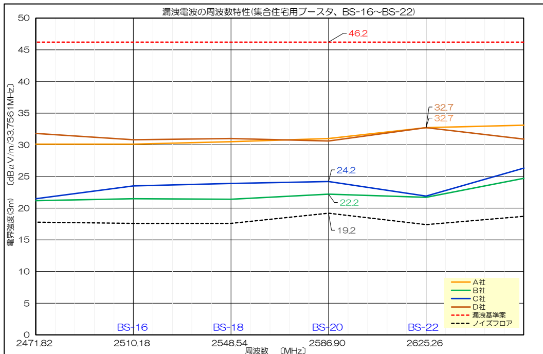
図 3. 6-10 集合住宅用ブースタの周波数特性 (2. 5GHz 帯)
