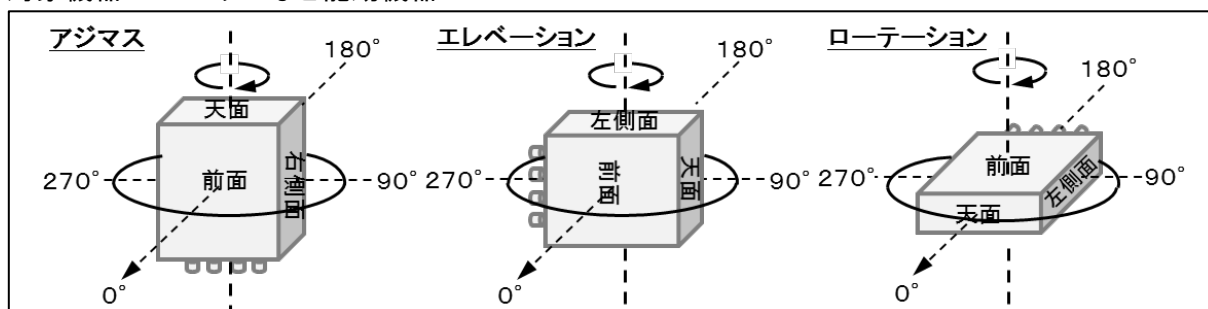
図 2.2 3 軸法の測定方向イメージ
