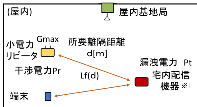
図 3.4.2-5 WiMAX 小電力レピータ・端末・屋内基地局の干渉評価モデル（屋内）
