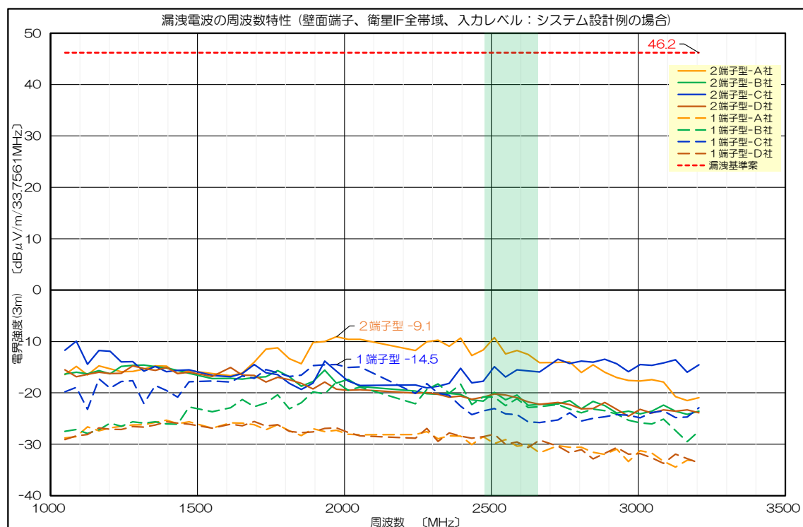
図 19 設計例に従って換算した場合の壁面端子の漏洩電波の最大電界強度
