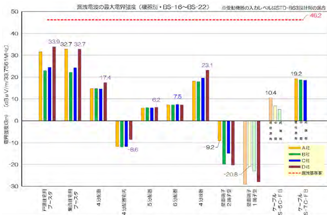
図 12 設計例に示された入力レベルに換算した場合の機器単体の漏洩電波の最大電界強度
