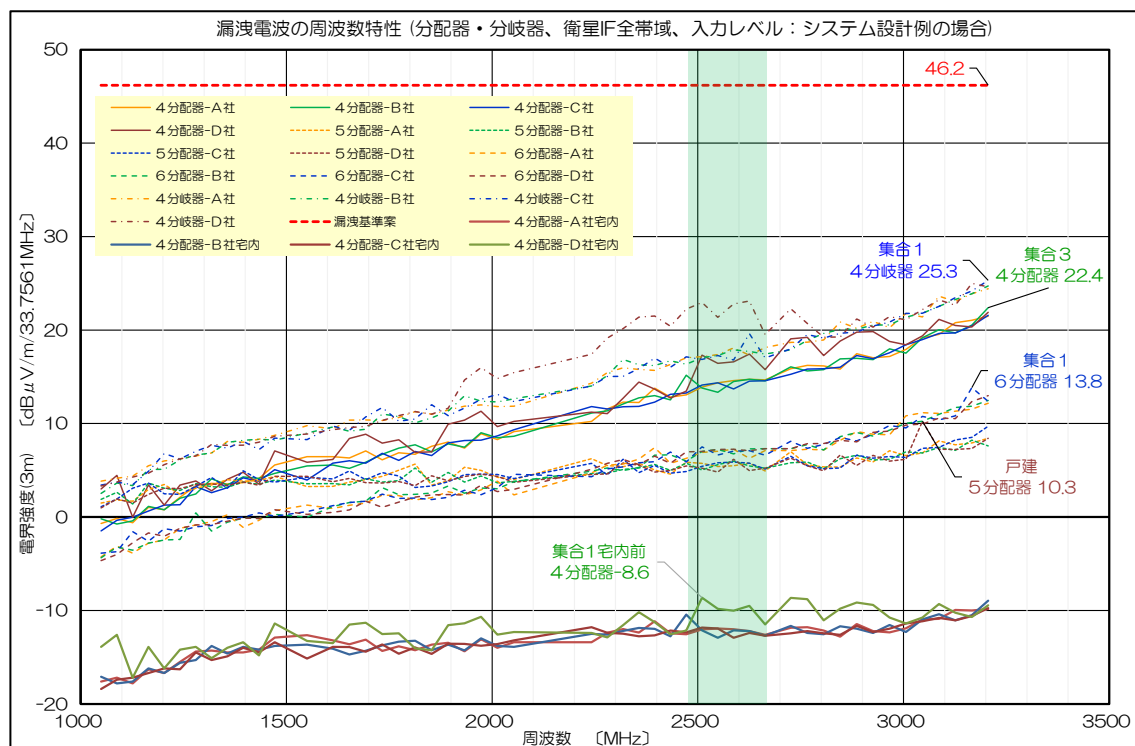
図 17 設計例に従って換算した場合の分配器・分岐器の漏洩電波の最大電界強度
