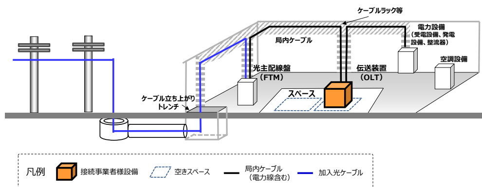
【図8-1 コロケーションのイメージ】
