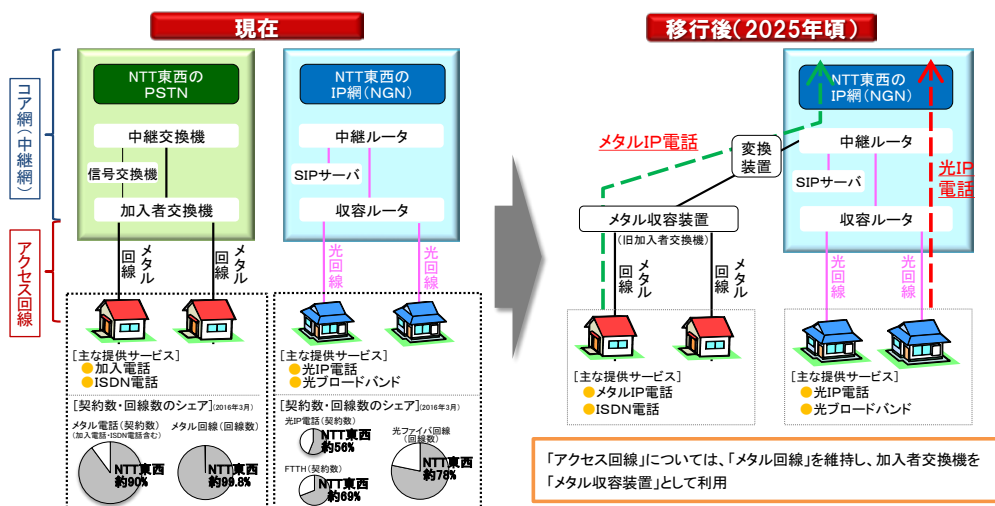
【図1-8 固定電話網からIP網への移行】
