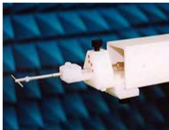
図 3.7 半波長ダイポールアンテナの外観
