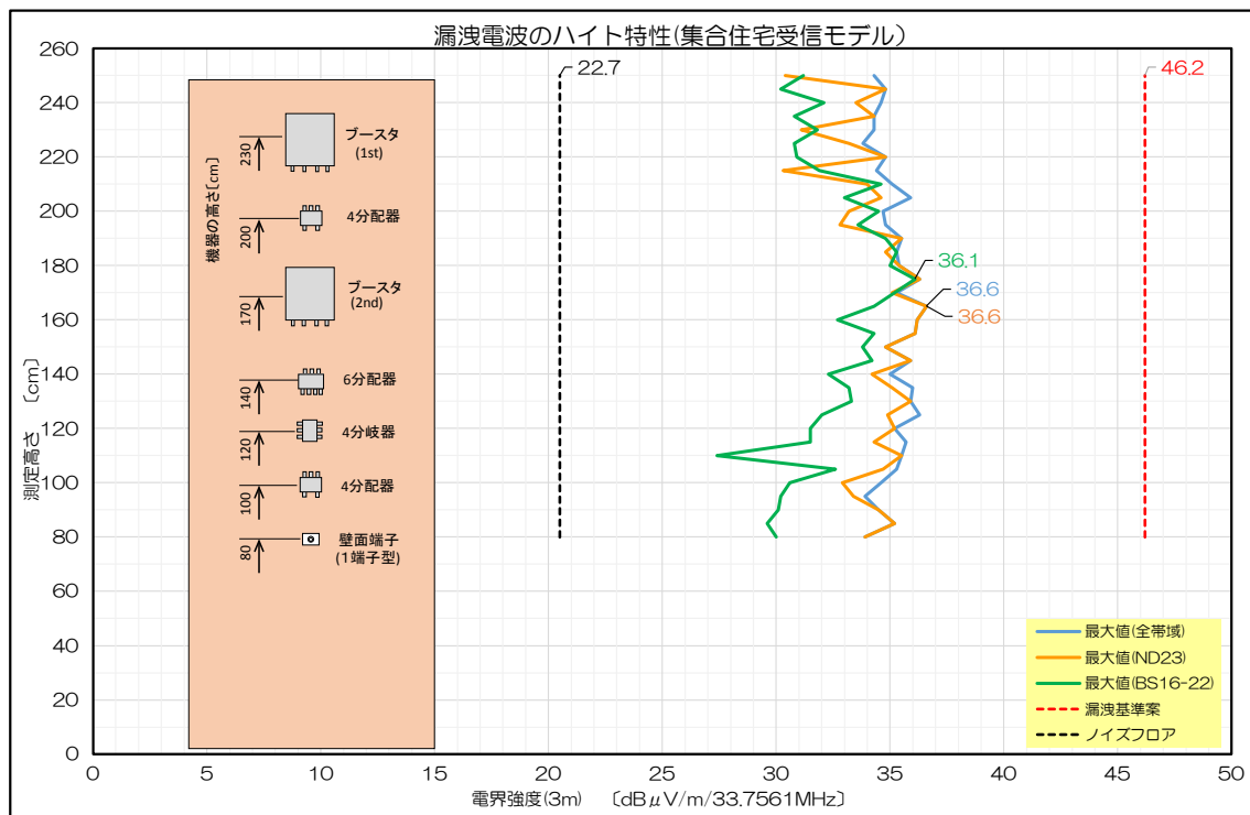
図 32 集合住宅モデルの漏洩電界強度の高さ方向の分布
