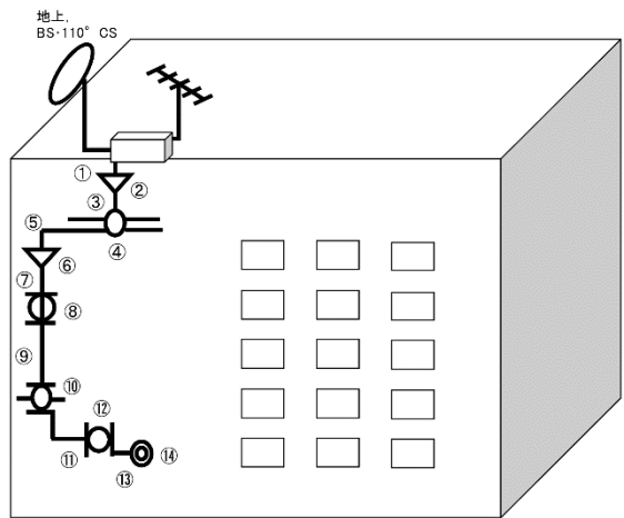
図 3.2-2 戸建住宅受信モデル
