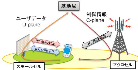
図 2. 4. 2-1 5Gの無線アクセスネットワーク
