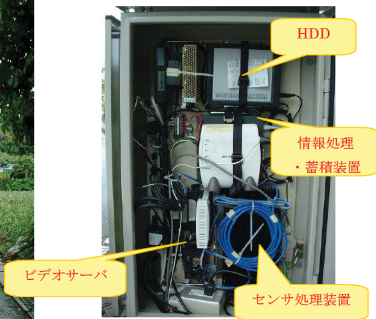
図 2-8 筐体内部写真
