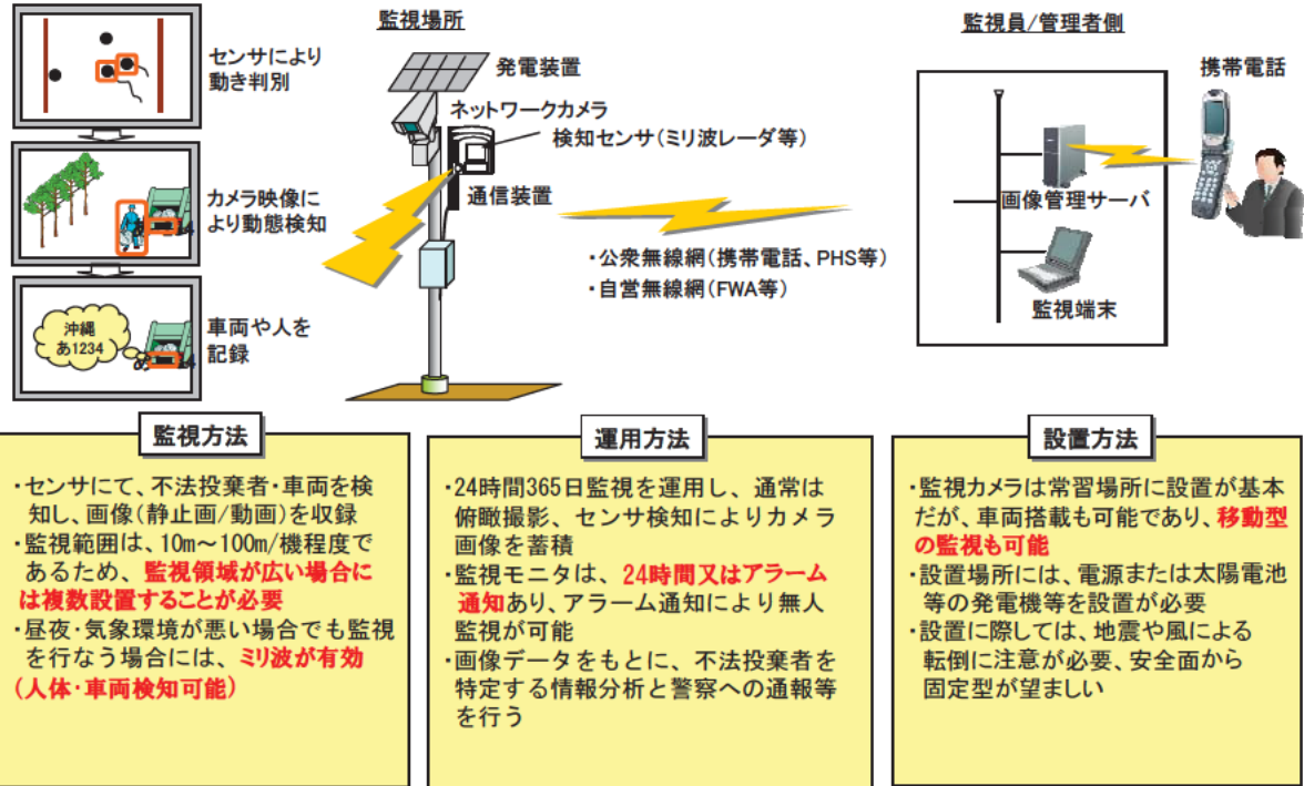
図 6-5 沖縄に適した不法投棄監視システム案 (平成 17 年度報告書より)
