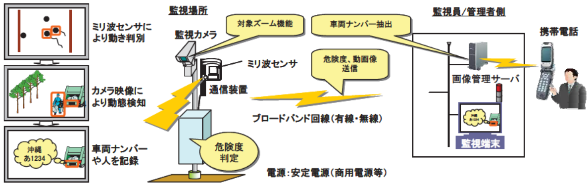
図 6-6 ミリ波センサを利用した不法投棄監視システム例
