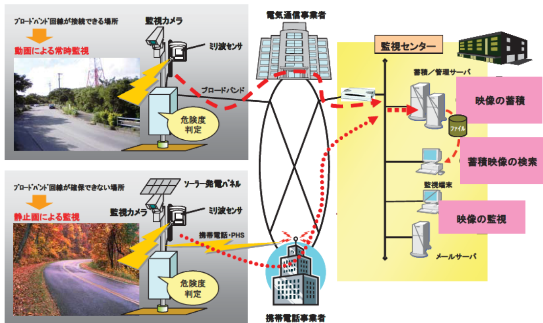
図 6-8 回線設定イメージ
