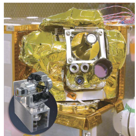
図2-9 光通信機器（SOTA）
