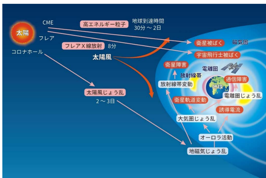
図3-13 宇宙天気現象の発生と障害
