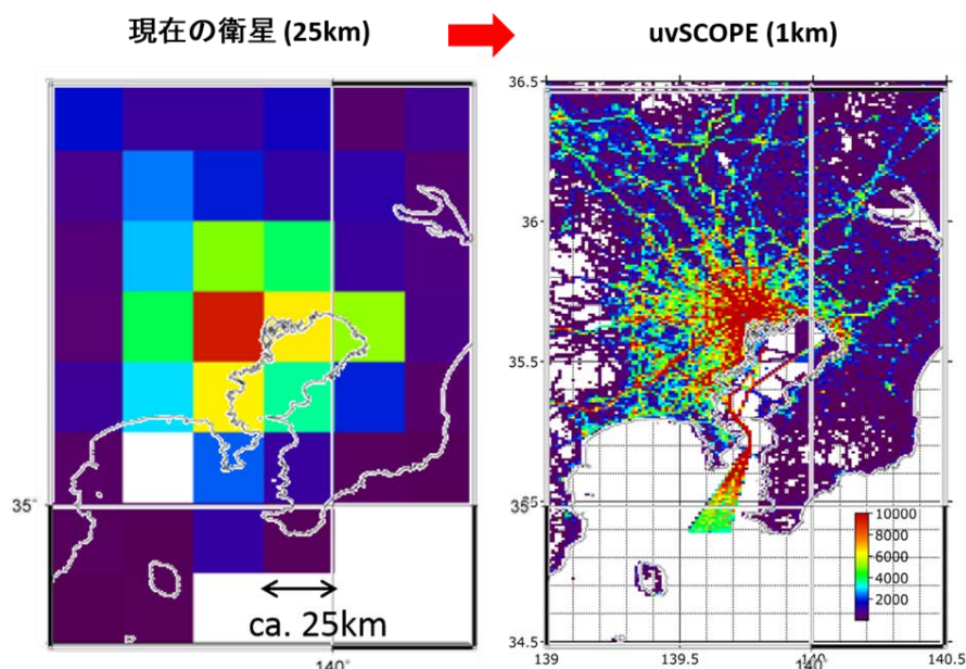
図 3 - 3 uvSCOPEによるNO 2 観測目標
