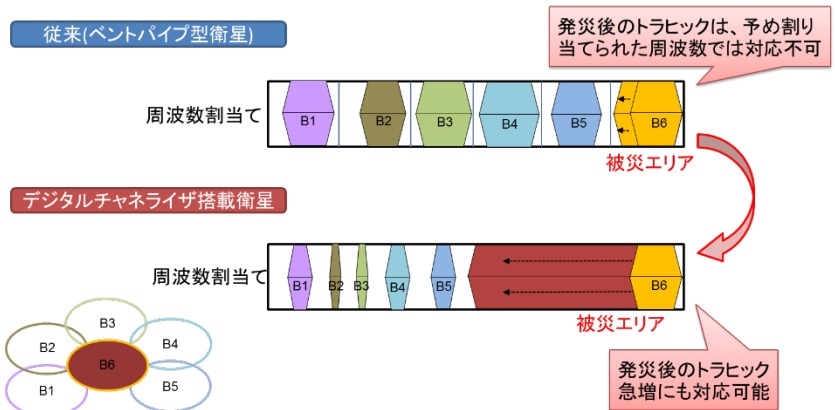
図2-7 デジタルチャネライザの概要
