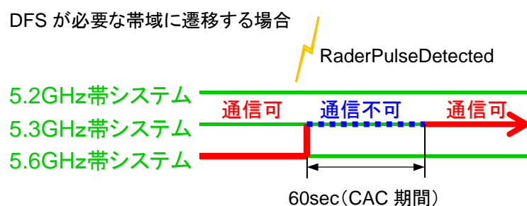
図 2.2.3-1 DFS 機能
