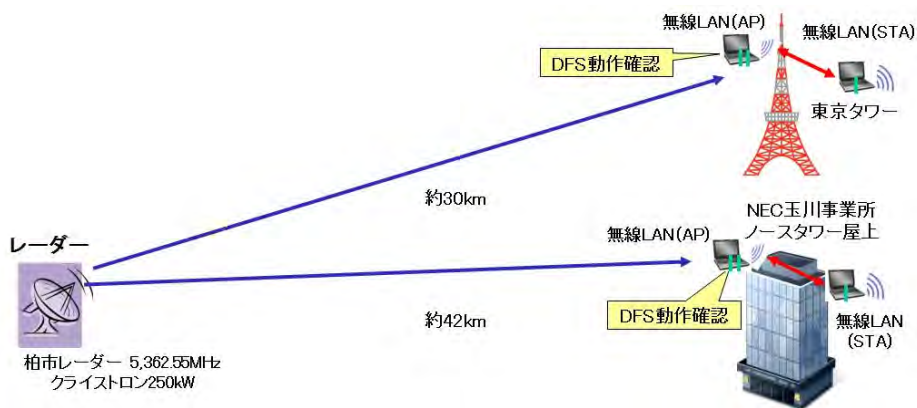
図 4.3.2.1-3 測定概要
