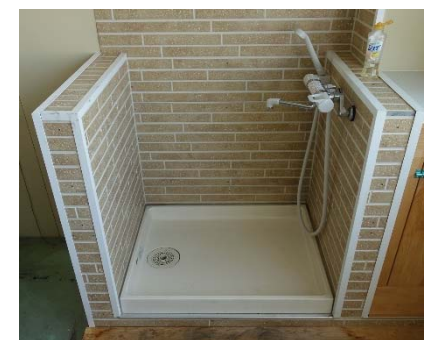
事業所が整備しているウドゥ用設備の例 (株)半谷製作所
