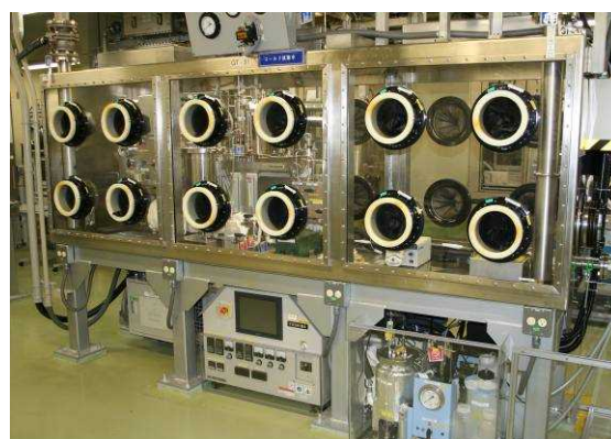
超臨界水有機溶液分解装置 (ROSE)
