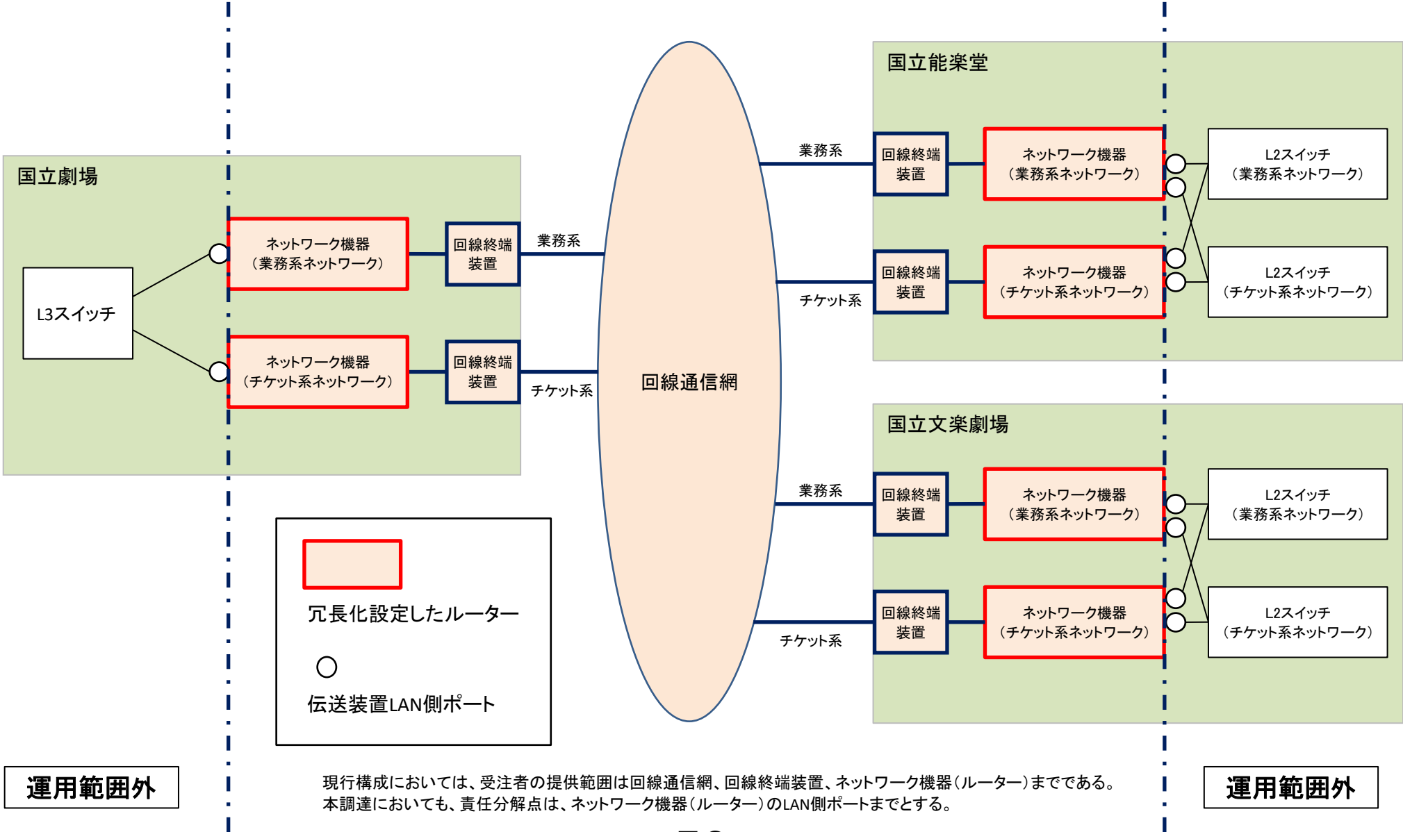
別紙2-3 現行振興会WAN構成図(1/2)
