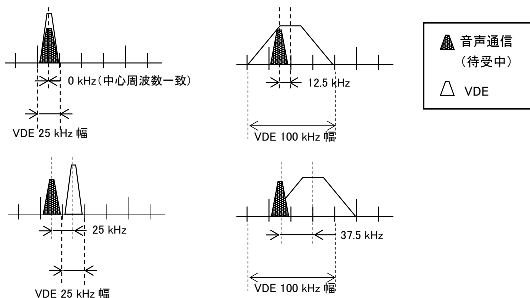
図 1.2.3 スケルチオープン測定検討条件模式図
