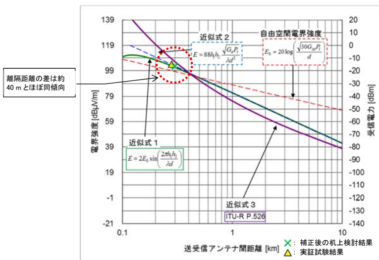
図 6.3-5 補正後の机上検討結果と実証試験結果の離隔距離の比較(試験項目 4) (16QAM 100 kHz、隣接チャネル干渉検討)
