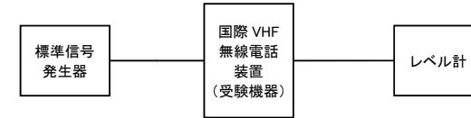
図 5.1-10 スケルチオープン測定検討のための試験系統図
