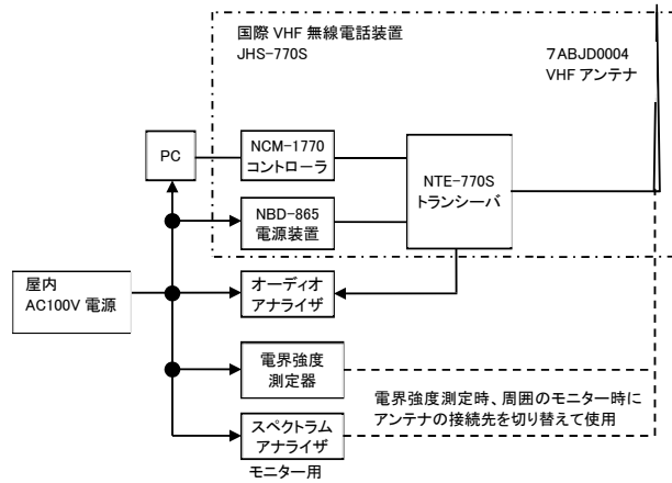
図 6.1-3 測定機器系統(海岸局)
