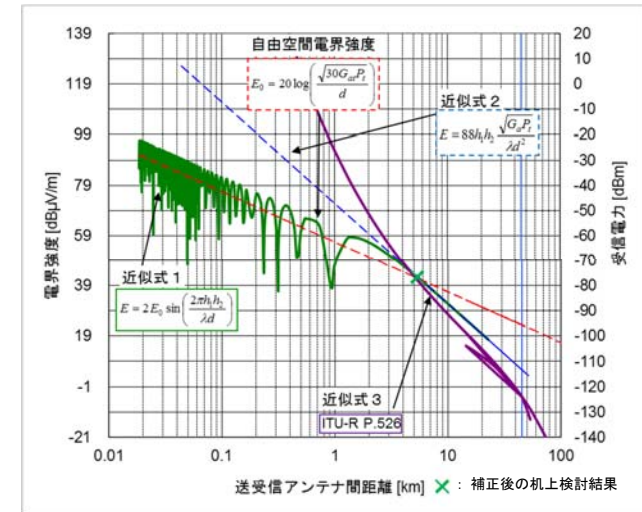
図 6.1-14 距離対受信電力(希望波 補正後の 8.9 mW 送信時)
