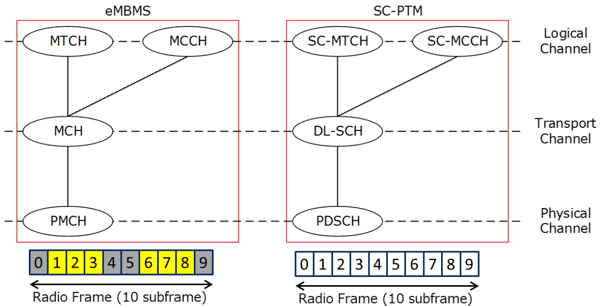
参考図 1-4 eMBMS と SC-PTM のチャンネルマッピングの比較
