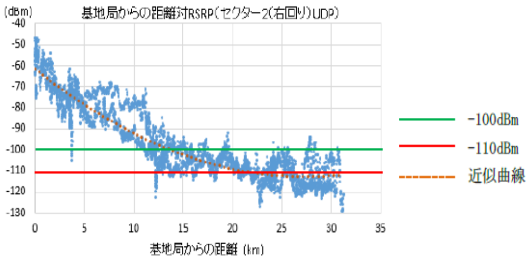
参考図 2-3 実験結果例-2 (基地局からの距離対 RSRP)
