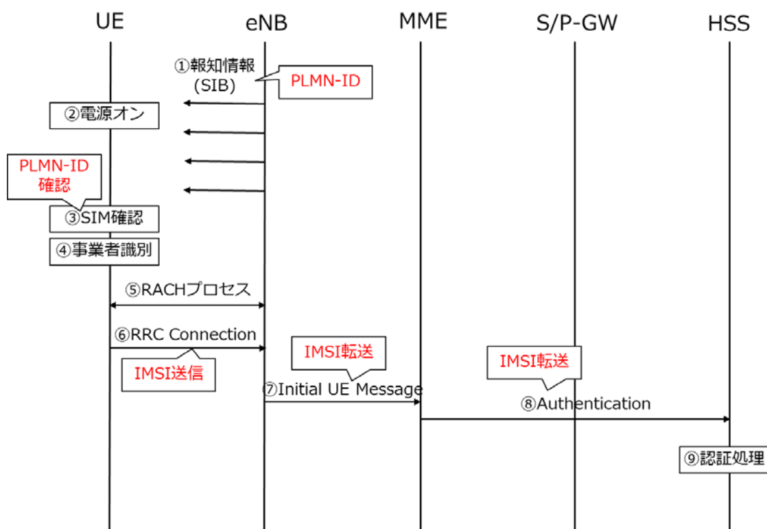
参考図 4-1 IMSI 認証プロセス例
