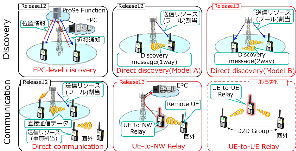
参考図 1-3 ProSe/D2D 機能
