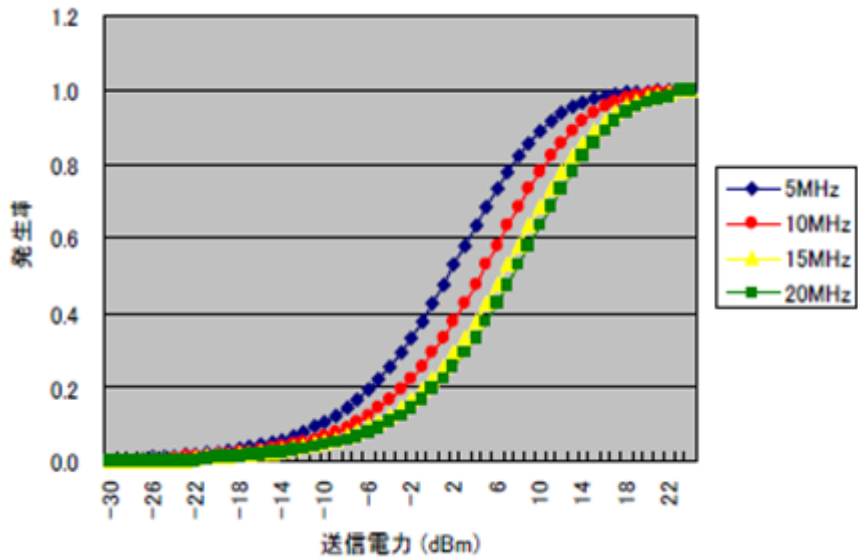
図 3-21 LTE 移動局の送信電力累積確率モデル(参考)
