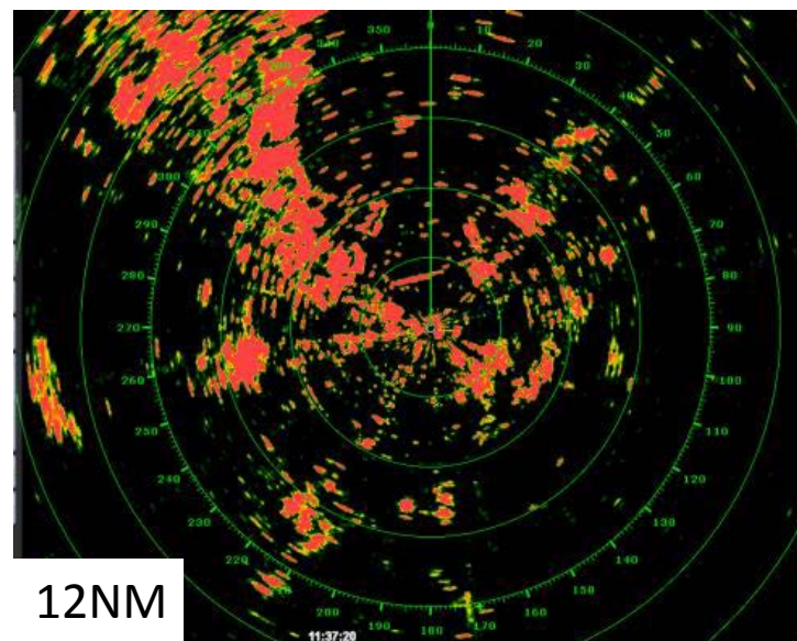
図-2 固体素子レーダー送信時の 固体素子レーダー映像 (干渉除去ON)
