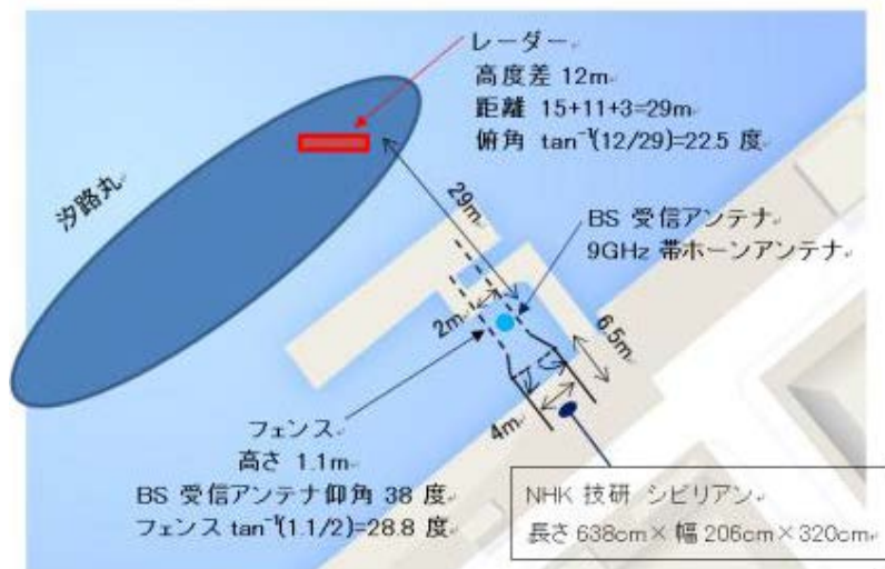
実験系統図
