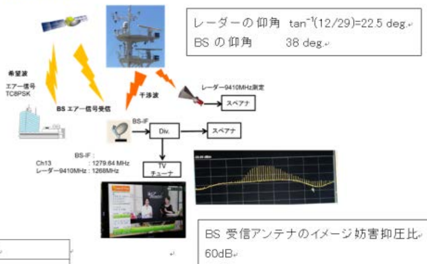
実験系統図
