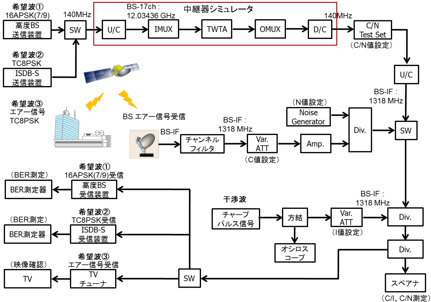
図1 干渉測定系統図
