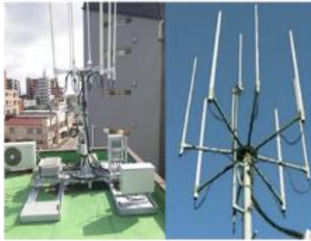
基地局(アンテナの例)
