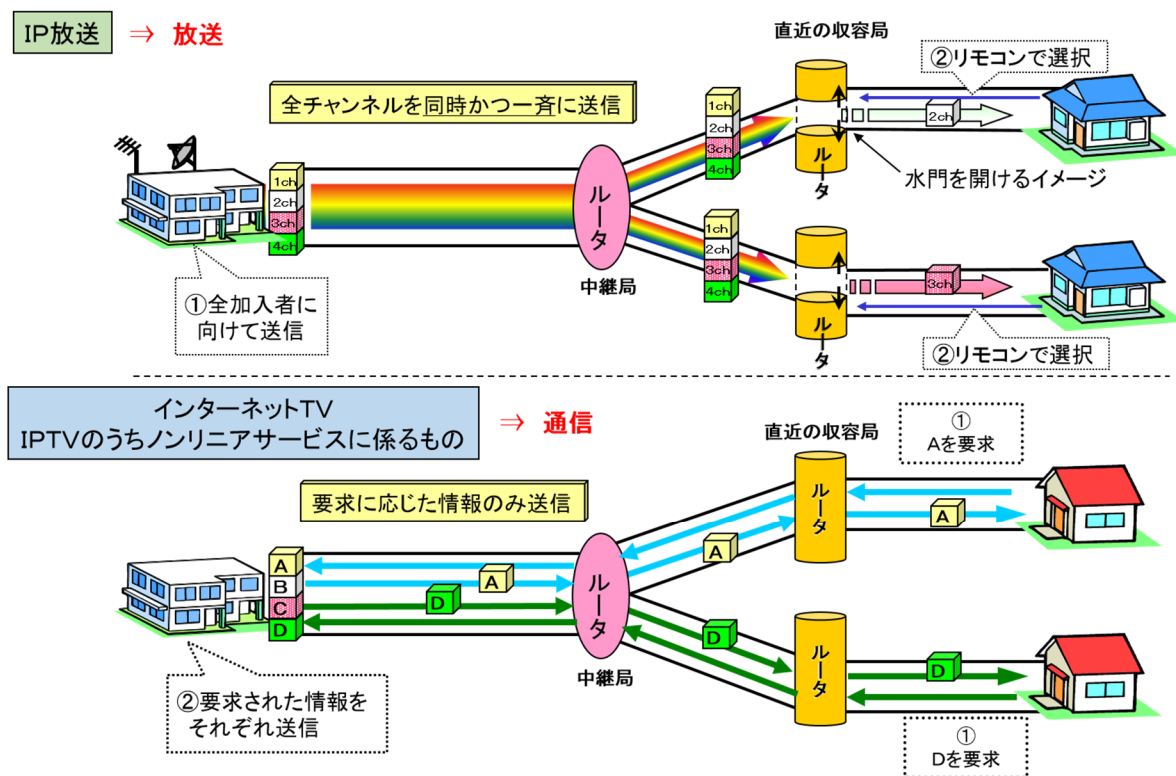
図 3.4 IP 放送のイメージ
