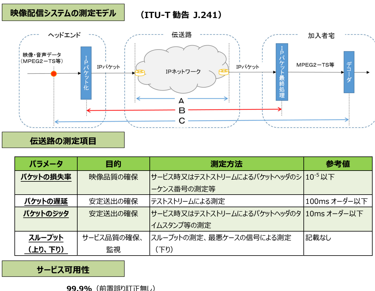
図 3.5 IP ネットワーク上で配信される映像に係る QoS と測定方法の事例
