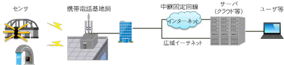
図 3.2 LPWA サービスのネットワーク構成イメージ
