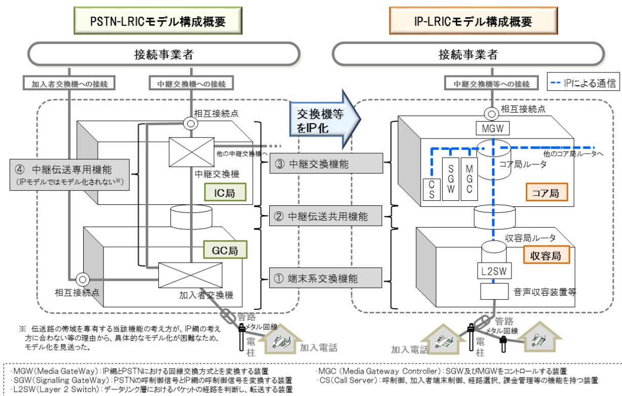
(図表 10 改良IPモデルの構成概要)
