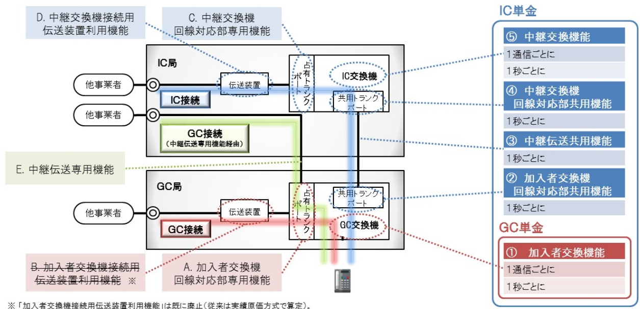
(図表 14 GC接続料とIC接続料の構成)
