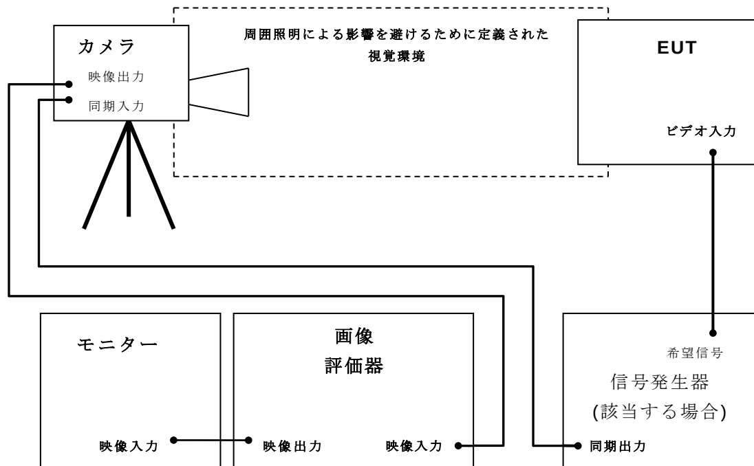
図 D.2 – ディスプレイで使用するためのビデオカメラシステムによる試験セットアップの例
