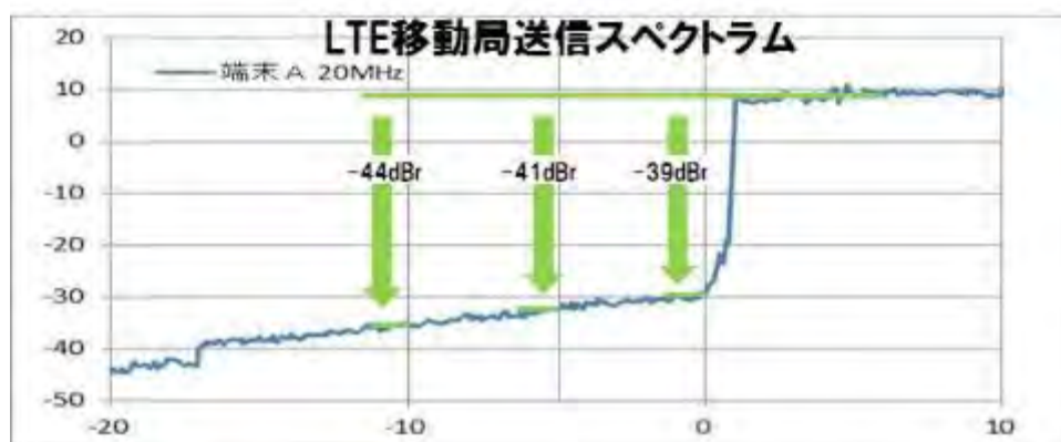
図参 2. 2. 1-3 LTE 移動局の送信スペクトラム例
