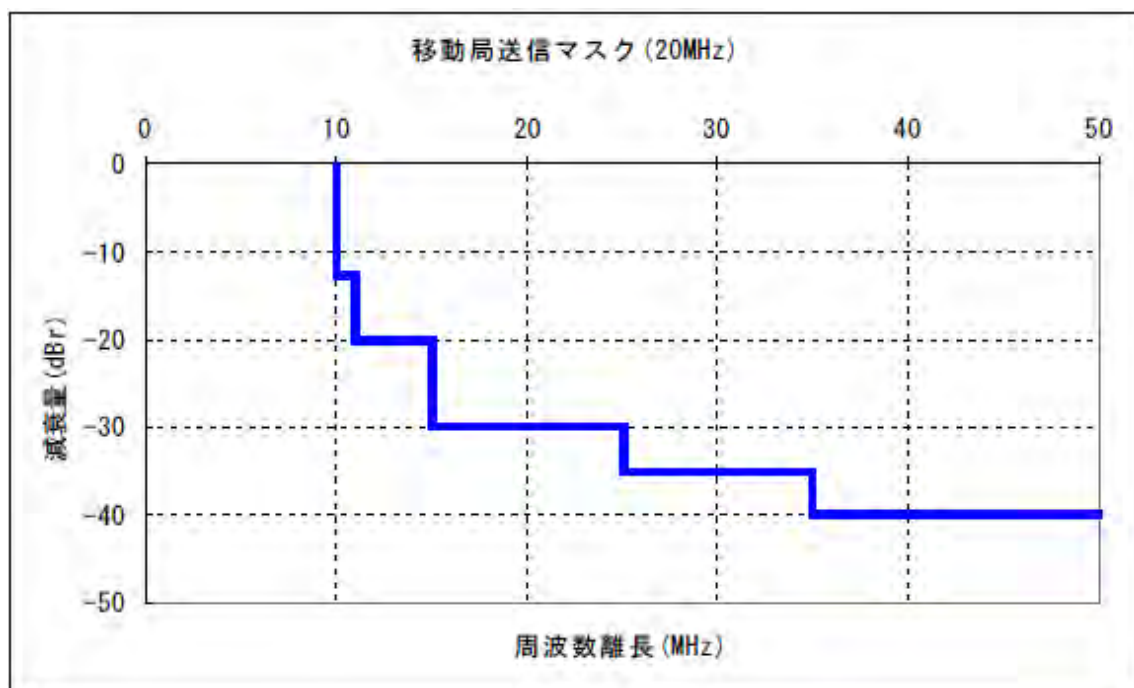
図参 1. 2-2 XGP 移動局送信マスク
