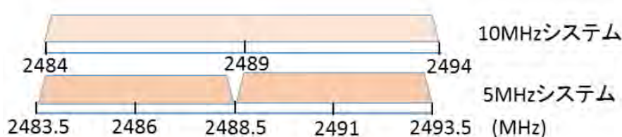
図 2. 2. 7. 1-1 ロボット用無線システムのチャネル配置
