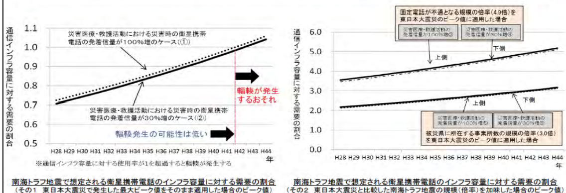
図1. 2-7 将来の大規模災害に備えた通信容量拡大
