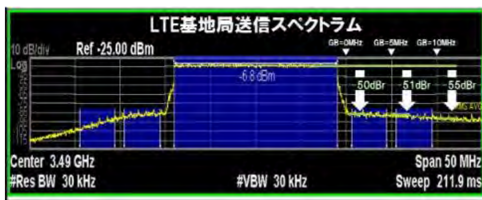
図参 2. 2. 1-2 LTE 基地局の送信スペクトラム例
