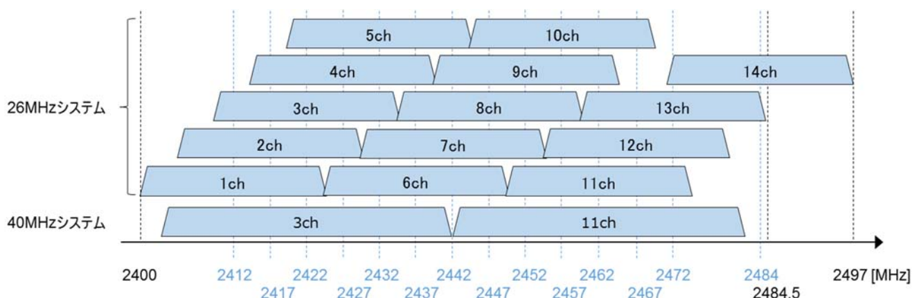
図4.1.1-2 2.4GHz帯無線LAN (802.11b/g/n) のチャンネル配置
