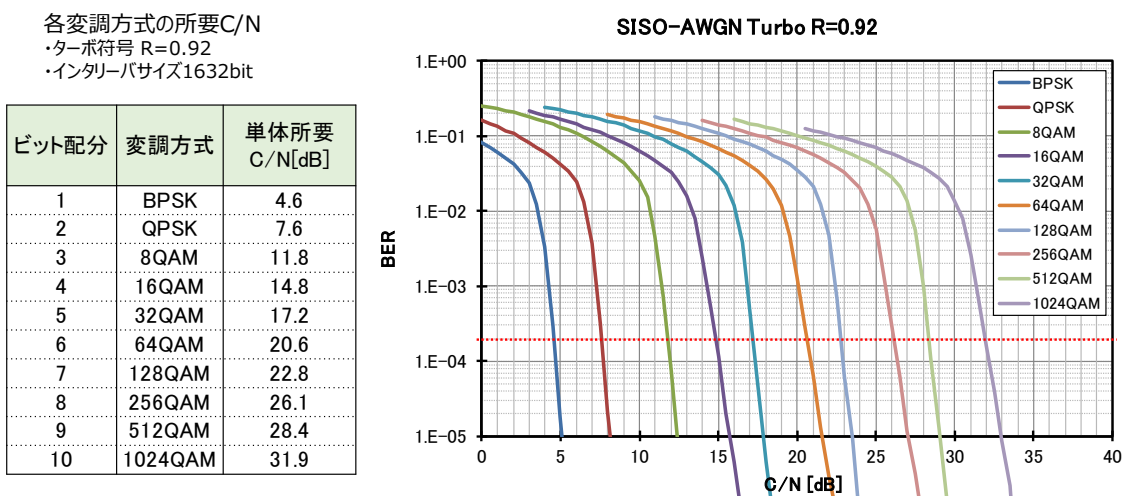
図 3-4 単体所要 C/N (R=0.92 の場合)
