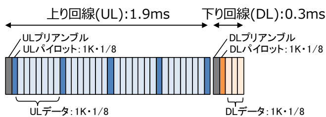
図 1-2 TDD フレーム構成
