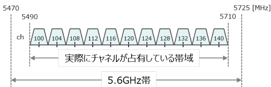
図2. 6. 1 5. 6GHz帯のチャンネル配置
