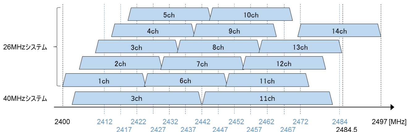
図4.1.1-2 2.4GHz帯無線LAN（802.11b/g/n）のチャネル配置
