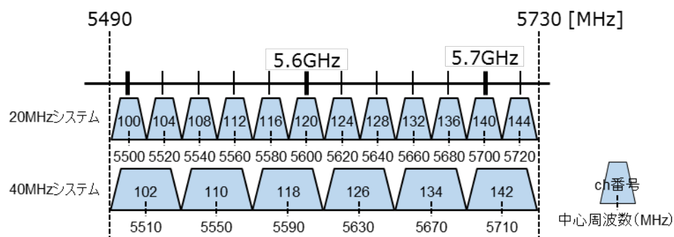
図 5.2.1 OFDM 以外の 5.6GHz 帯小電力データ通信システムのチャネル配置
