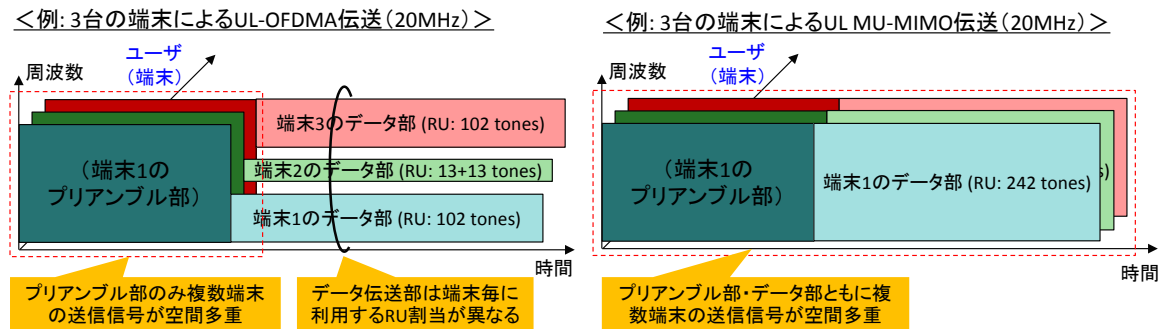
図4. 2. 3. 1 UL-OFDMA及びUL MU-MIMO伝送における無線フレームの空間多重
