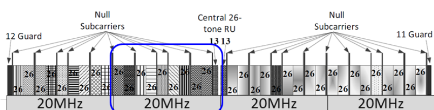
(↑左図はこの部分に着目) 802.11axのRU配置* (160MHzのうちの80MHz分)
