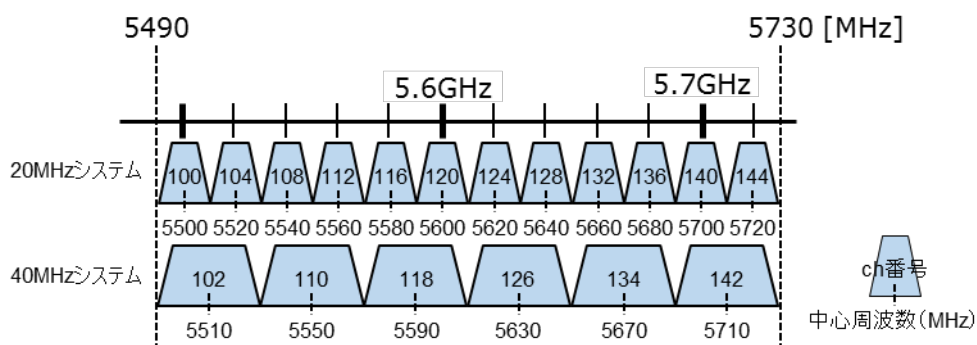
OFDM 以外の 5.6GHz 帯小電力データ通信システムのチャンネル配置
