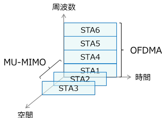
図2.5.3-2 802.11axで導入するマルチユーザ伝送技術
