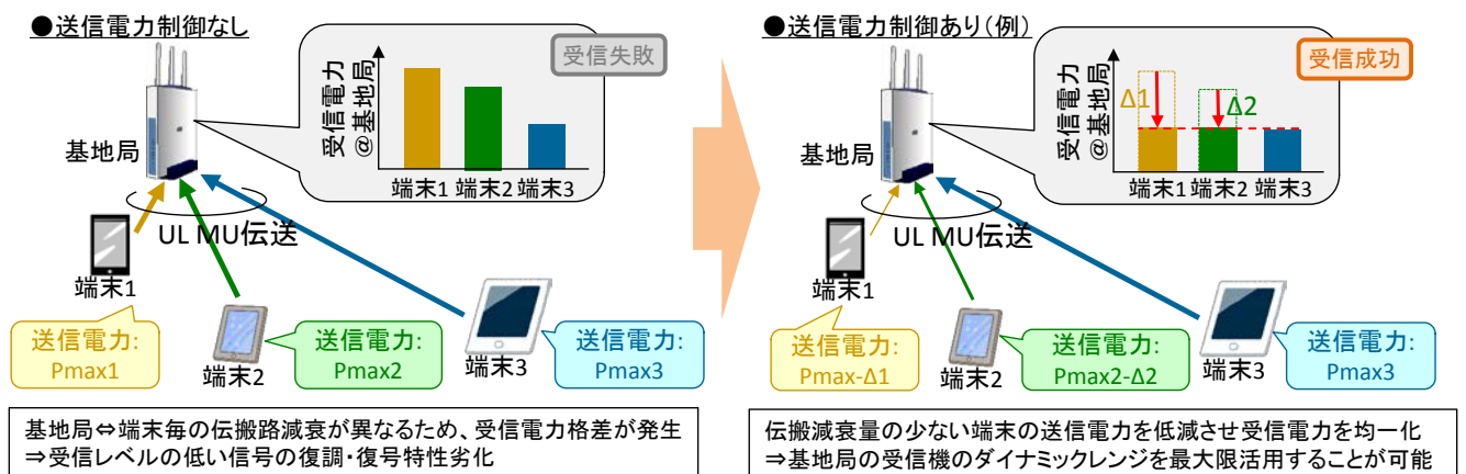
図4. 2. 3. 2 UL MU伝送における送信電力制御の概要
