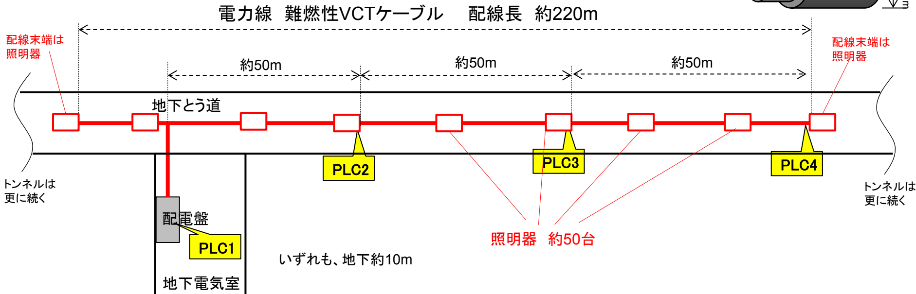
上面図
