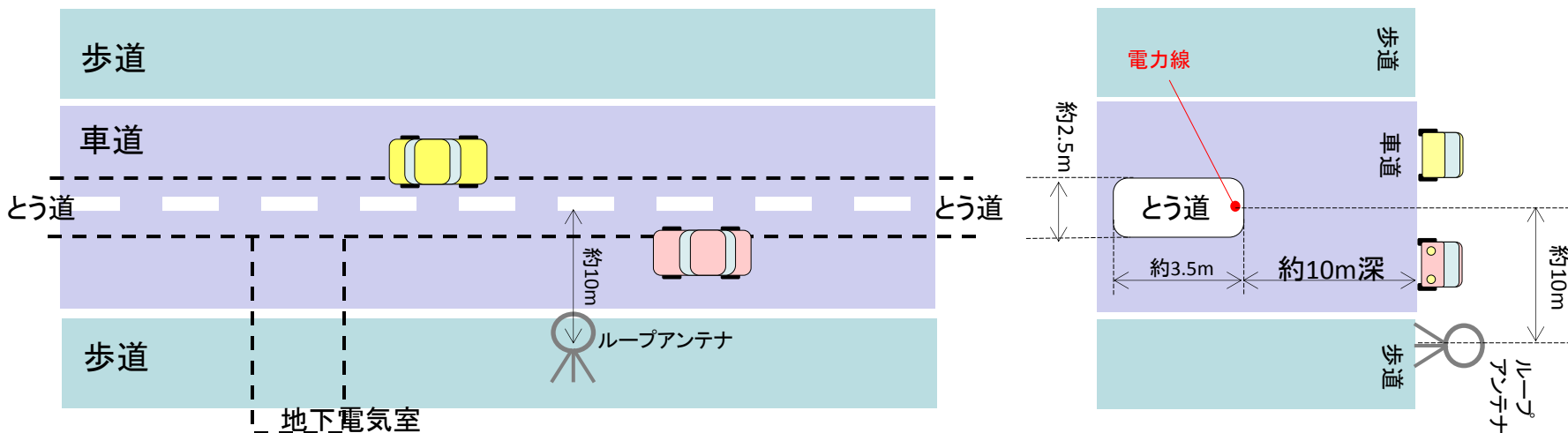
上面図
