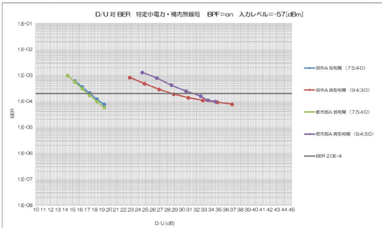
図 12-2 特定小電力・構内無線局からの被干渉における D/U 対 BER
