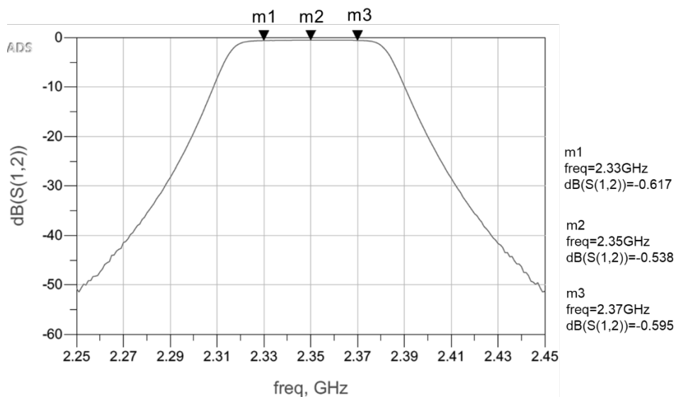
図 10-4 受信部内蔵 BPF 特性
