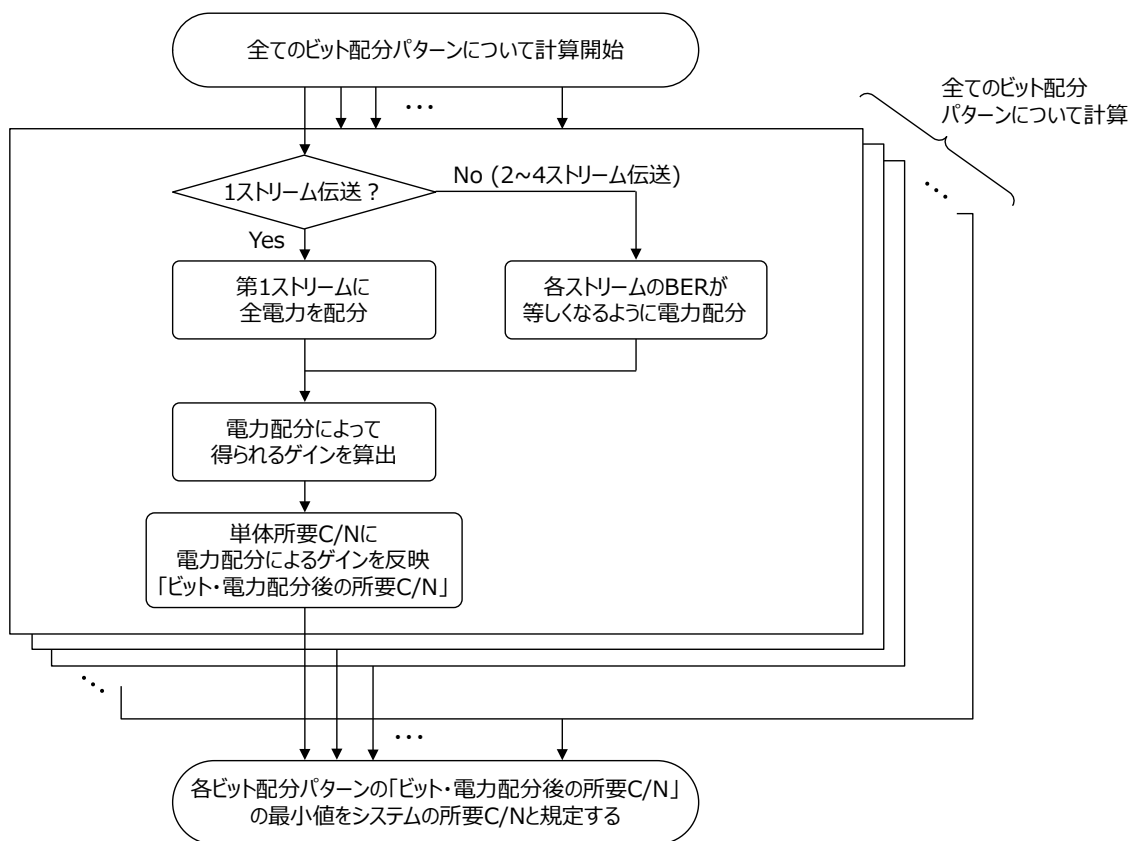
図 3-10 所要 C/N 算出のフローチャート
