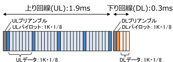
図2-1 TDD フレーム構成
