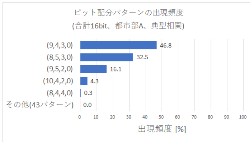
図9-5 ビット配分の出現頻度（その2）
