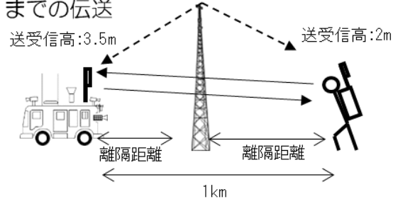
図 14-3 アマチュア無線局から 4K・8K 用 FPU への干渉モデル
