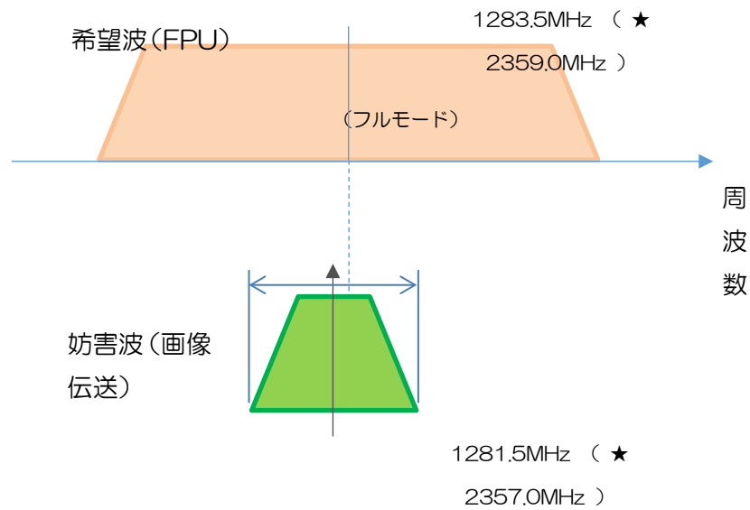
図 13-1 希望波と妨害波の周波数配置 (実験は 2.3GHz 帯内)
