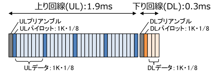
図 1-5 TDD フレーム構成
