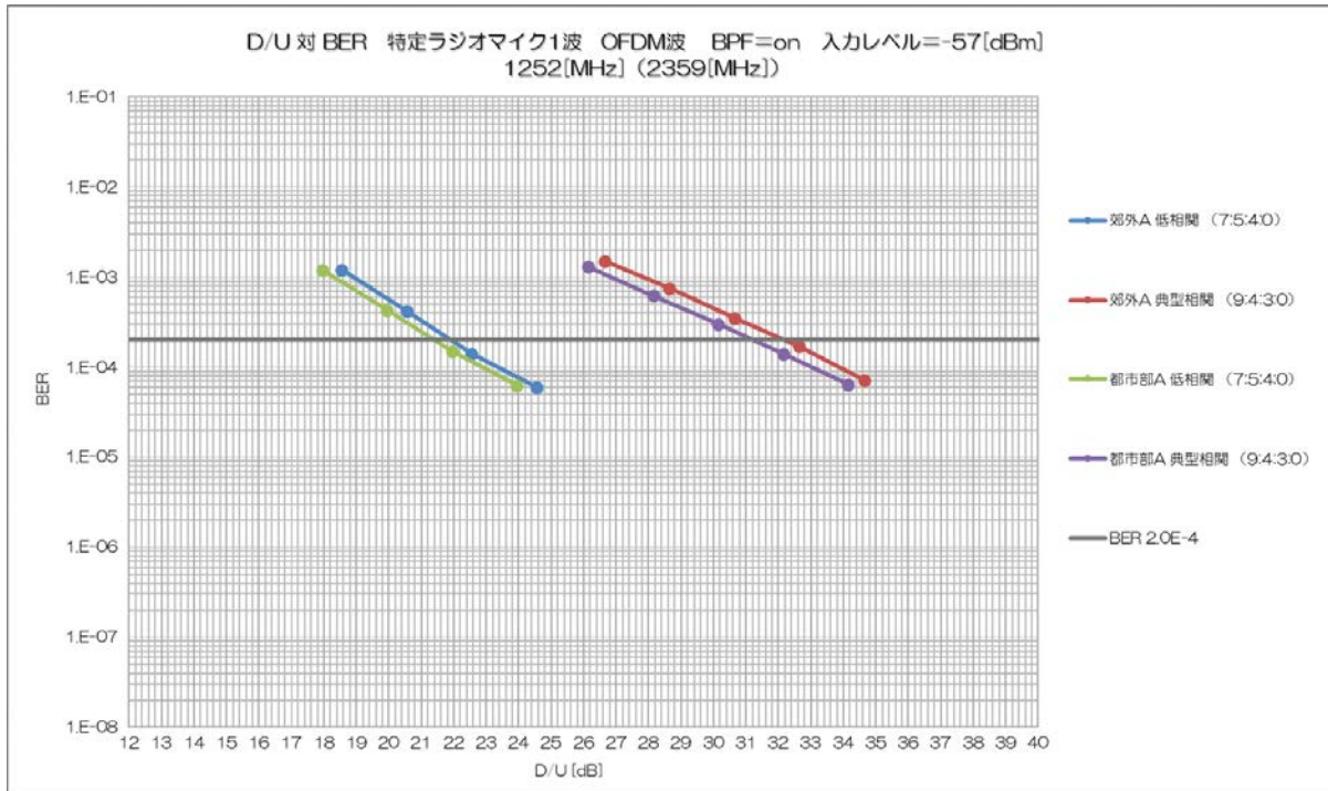
図 11-8 デジタル (OFDM) RM 1 波の場合の D/U 対 BER
