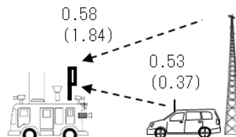
図 14-6 (参考) 現行 FPU とアマチュア無線移動局との離隔距離 (km)
