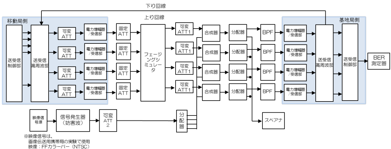
図 9-3 室内実験の構成図
