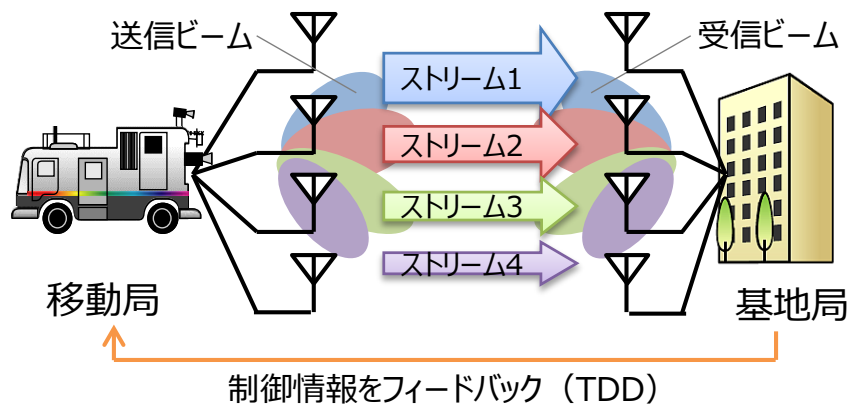
図2 SVD-MIMO技術のイメージ
