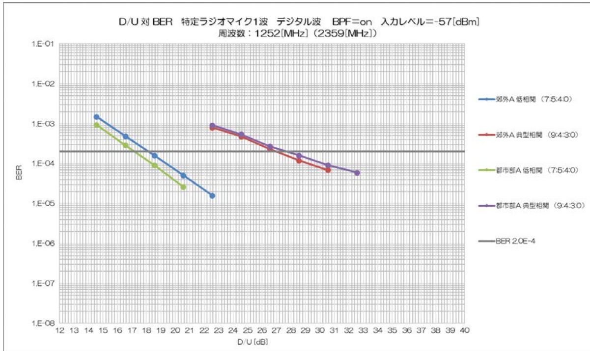
図 11-6 デジタル (DQPSK) RM 1 波の場合の D/U 対 BER
