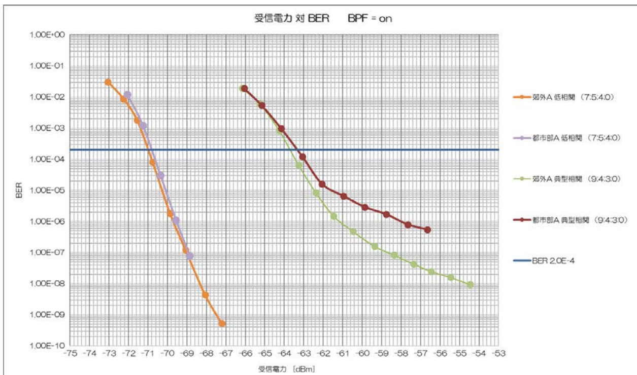
図 10-2 4\text{K}\cdot 8\text{K} 用 FPU の受信電力に対する誤り率特性
