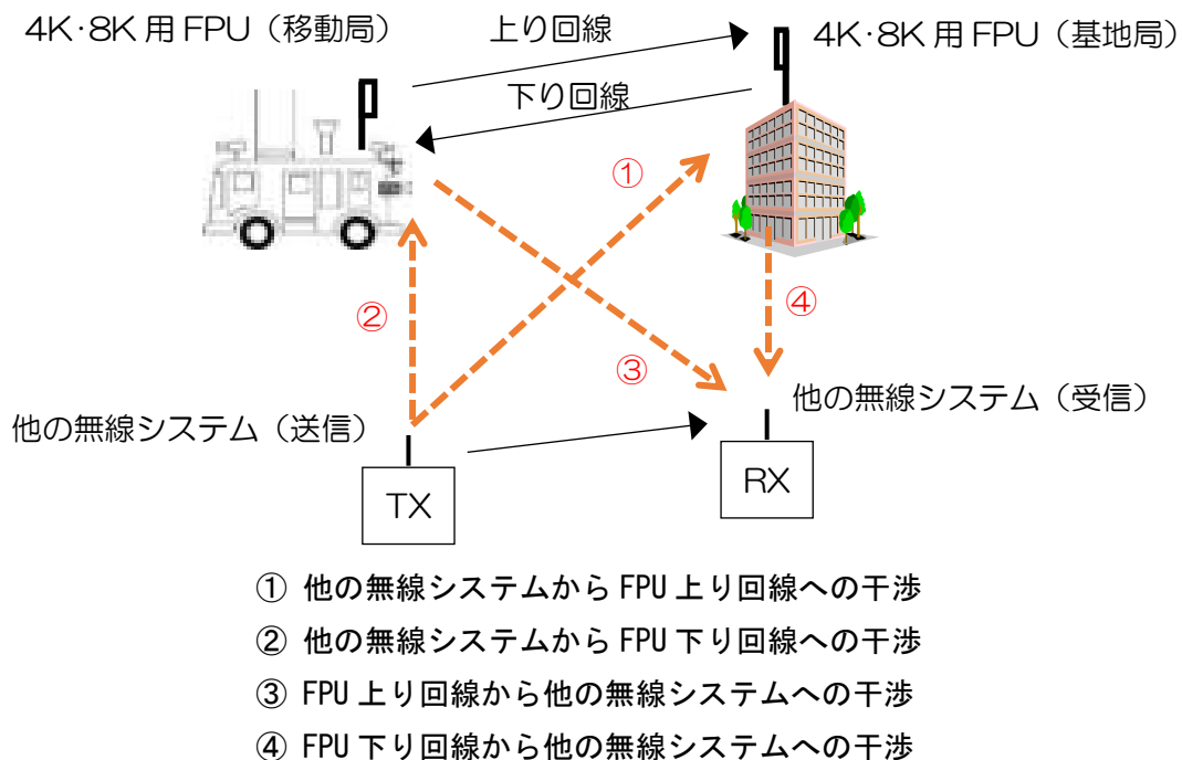
図8 干渉の組合せ
