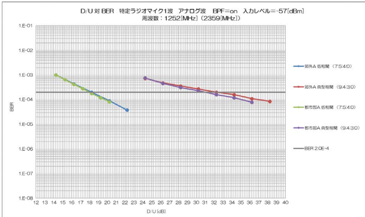
図 11-4 アナログ RM 1 波の場合の D/U 対 BER
