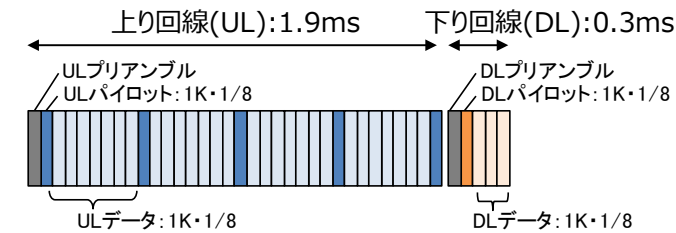
図 1-6 TDD フレーム構成
