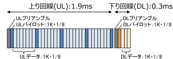
図 1-1 TDD フレーム構成
