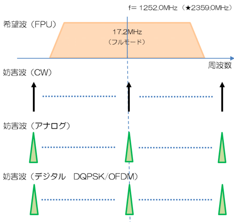
図9 妨害波1波と希望波の周波数配置
