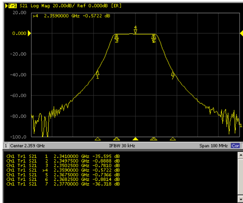
図 10-3 FPU 受信フィルタ特性の例
