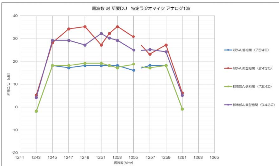
図 11-5 アナログ RM1 波の場合の周波数 対 所要 D/U
