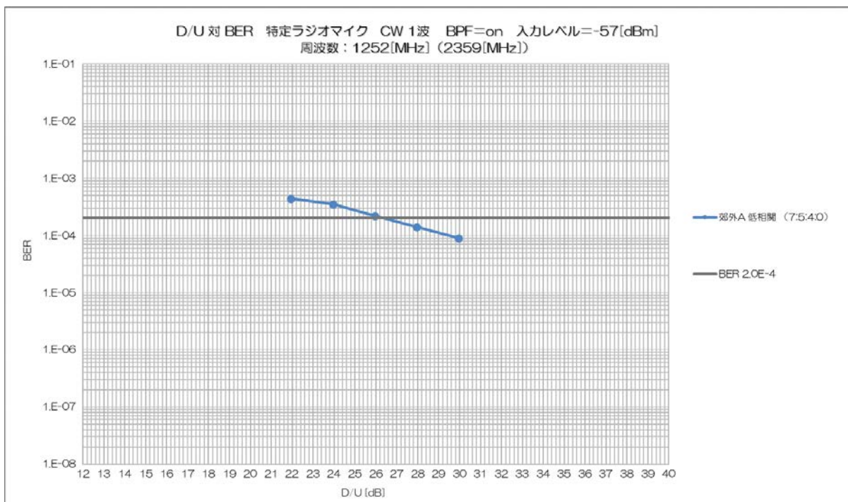
図 11-2 特定ラジオマイク (CW 1 波) からの被干渉における D/U 対 BER
