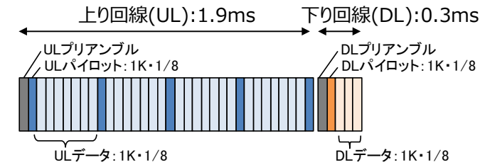
図 1-2 TDD フレーム構成
