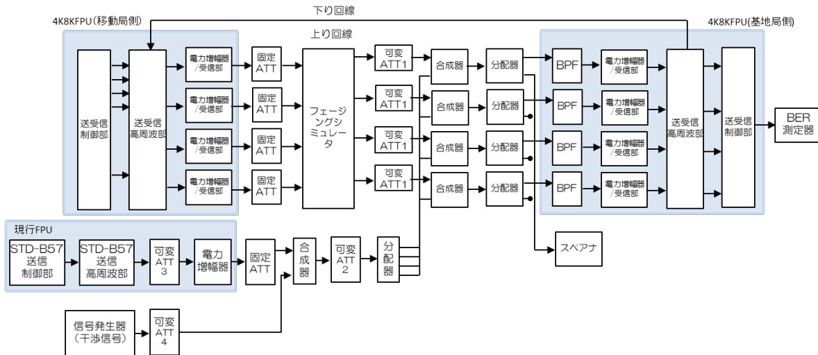
図 10-5 試験系統図
