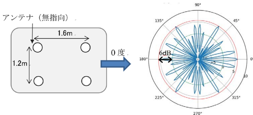
(a) 送信アンテナの配置例
