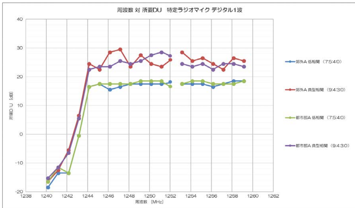
図 11-7 デジタル (DQPSK) RM 1 波の場合の周波数 対 所要 D/U
