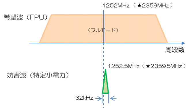
図 12-1 希望波と妨害波の周波数配置
