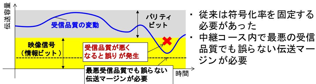
(a) 符号化率を固定する場合
