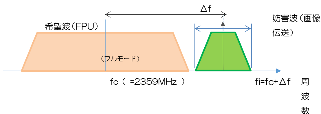
図 13-3 所要 D/U 測定における希望波と妨害波の周波数配置
