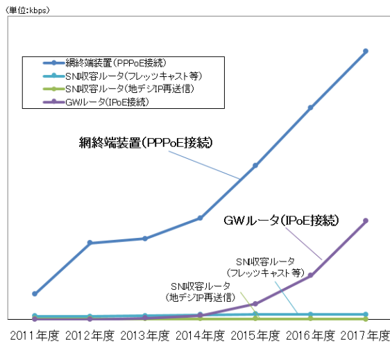
【図3-3 関門系ルータにおける実績トラフィック(総量)のトレンド】
